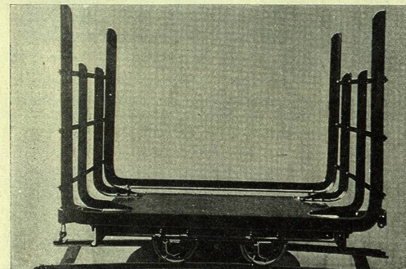
MODELO DE WAGONETA DECAUVILLE
