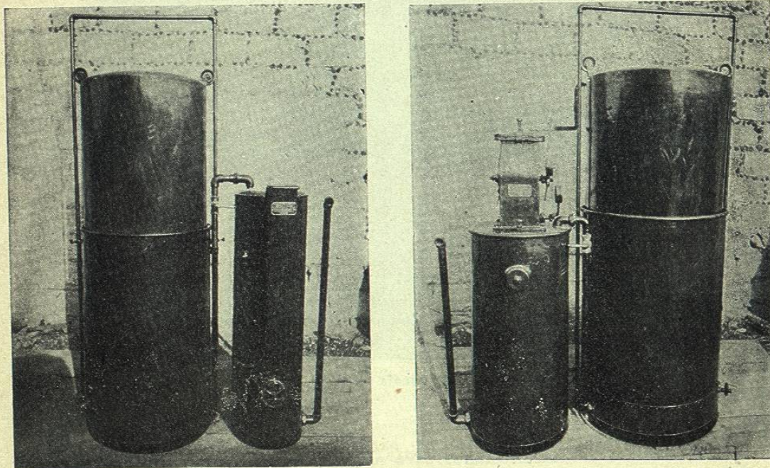
MODELOS DE APARATOS PRODUCTORES DE GAS ACETILENO
