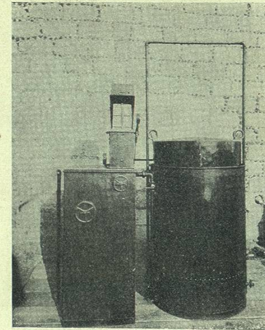
GENERADOR PARA GAS ACETILENO
