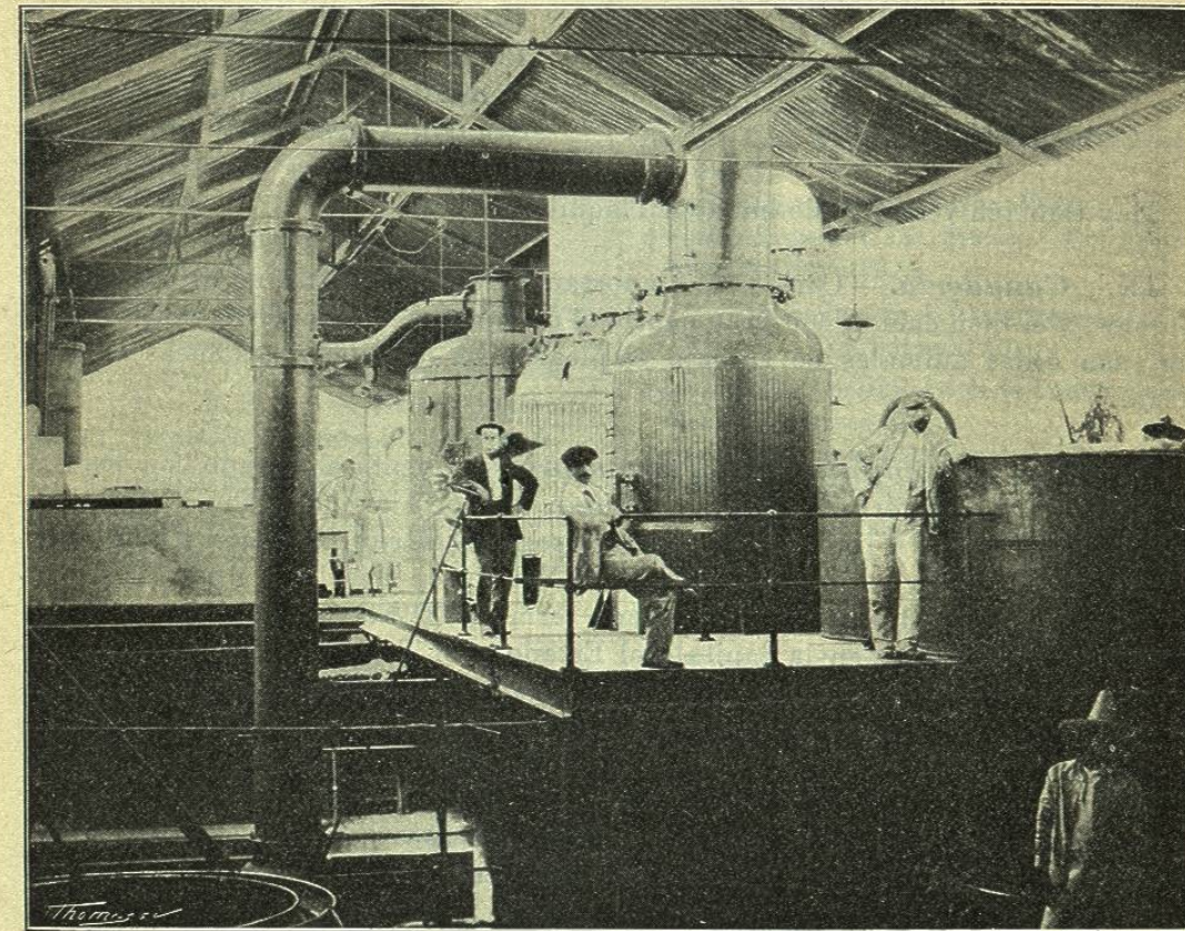
TACHO AL VACÍO EN LA «HACIENDA SANTA INÉS»
