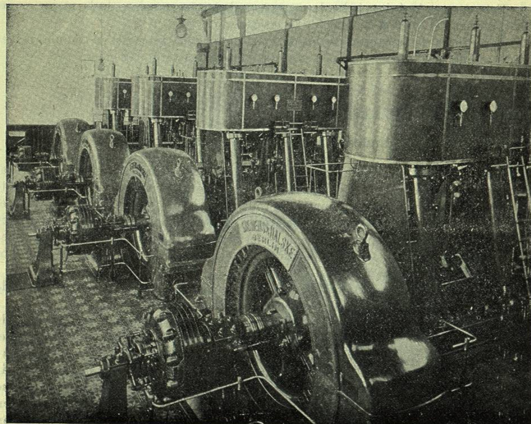
DINAMOS EN LA PLANTA ELÉCTRICA SIEMENS Y HALSKE
