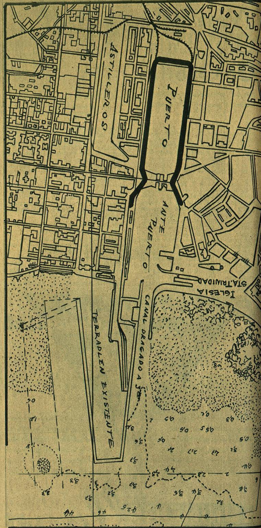
Plano del puerto de Cherbourg. La raya gruesa representa un muro alrededor del puerto. La compuerta que comunica con el antepuerto está abierta solamente una hora antes de la marea alta, y cerrada una hora después. No se abre durante la noche, entre las 20 horas y las 4.
