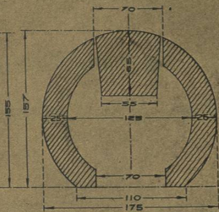
CORTE TRANSVERSAL SEGUN a-b
