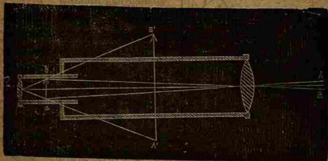
Teoría del aumento del anteojo.
