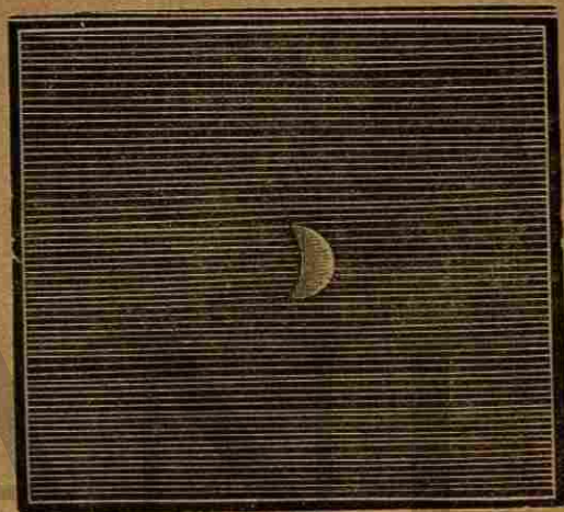
Aspecto del planeta Mercurio en su cuadratura.
