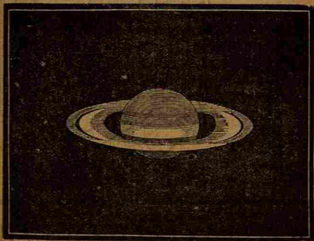
El planeta Saturno.
