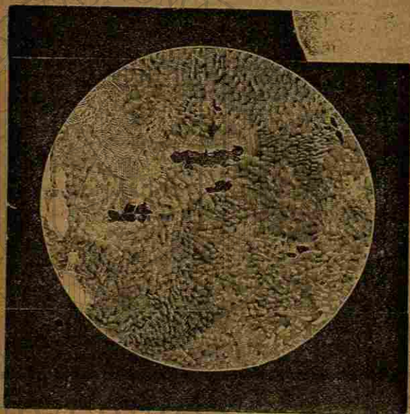
El Sol y sus manchas:
