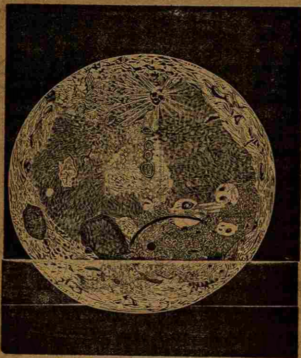
Carta topográfica de la Luna.
