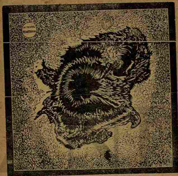
Tipo de mancha solar (14 Octubre 1883).
