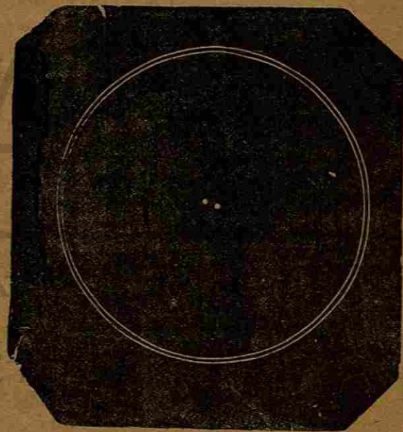
La estrella doble de la Virgen.
