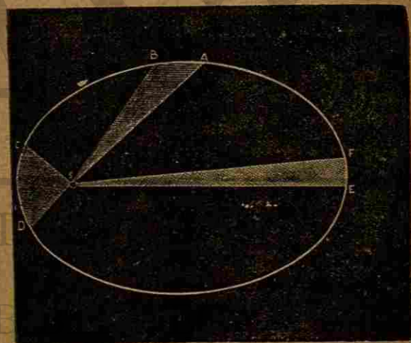
Explicación de los movimientos de los planetas.—Ley de las áreas.
