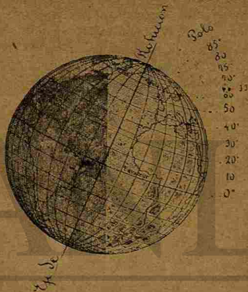
Inclinación de la Tierra.
