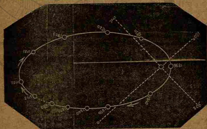
Órbita de la estrella doble de la Virgen.
