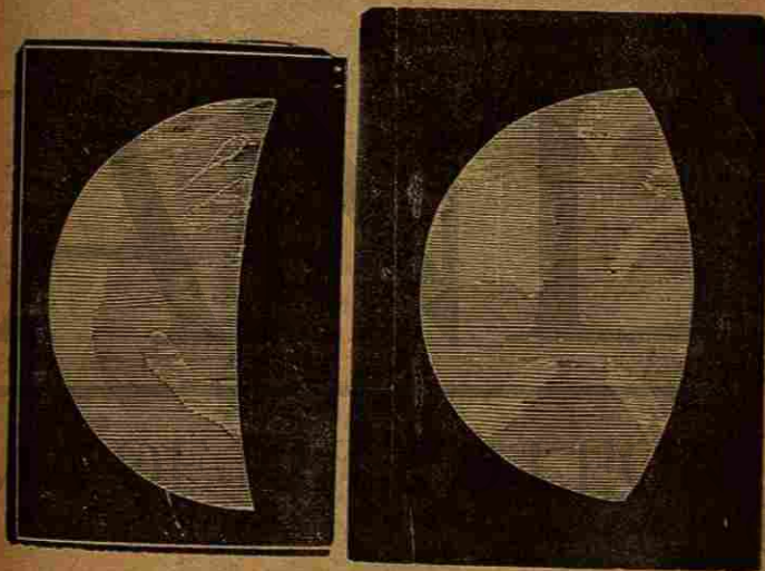
Vistas telescópicas de Venus.
