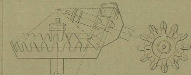
Engrenage de Roues d'angles.
