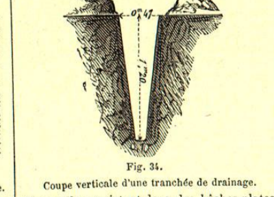
Fig. 34. Coupe verticale d'une tranchée de drainage.
