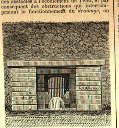
Fig. 32. Vue d'une bouche d'évacuation d'un collecteur de drainage.
