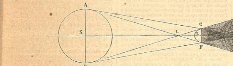
Fig. 3. Les éclipses de lune sont produites par l'intersection de la lune entre le soleil et la terre. Lorsque la terre entre dans le cône d'ombre projetée par la lune, les points de sa surface qui sont plongés dans cette ombre ne reçoivent plus les rayons du soleil et se trouvent dans une obscurité complète.
