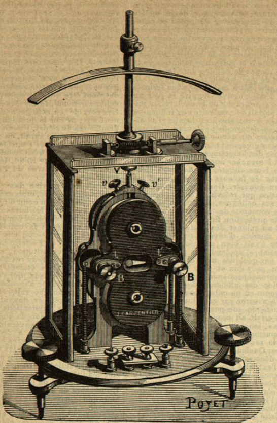
Fig. 1. — Galvanomètre de Thomson.
