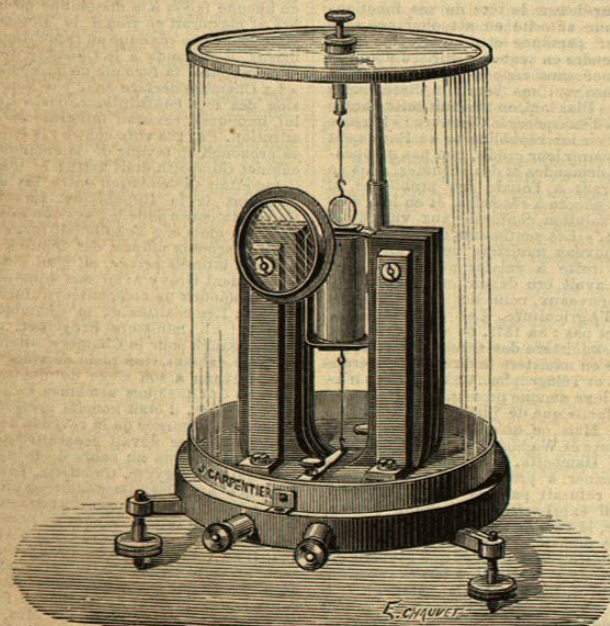
Fig. 2. — Galvanomètre aperiédrique de MM. Deprez et d'Arsonval.
