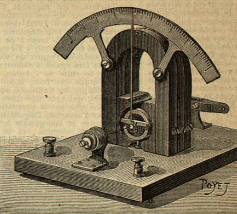
Fig. 3. — Galvanomètre de MM. Deprez et d'Arsonval.
