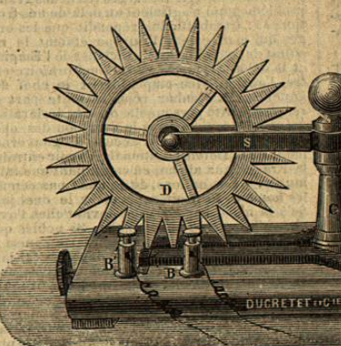
Fig. 1. — Roue de Barlow.
