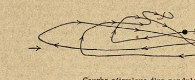
Courbe sismique d'un pendule libre.
