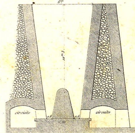
Horno para yeso.
