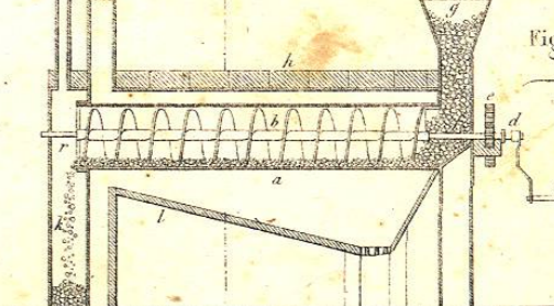
Horno para yeso.
