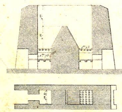
Horno para puzolana
