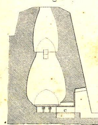
Horno de cal á fuego periódico.
