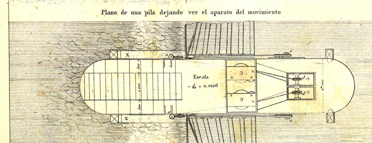
Plano de una pila dejando ver el aparato del movimiento
