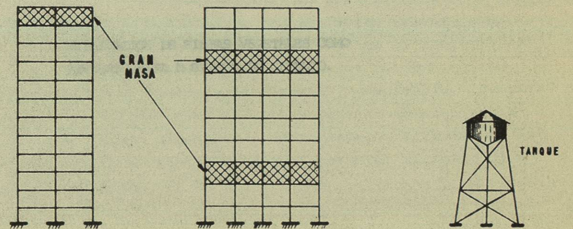
FIGURA 6b - DISTRIBUCION IRREGULAR DE MASAS
