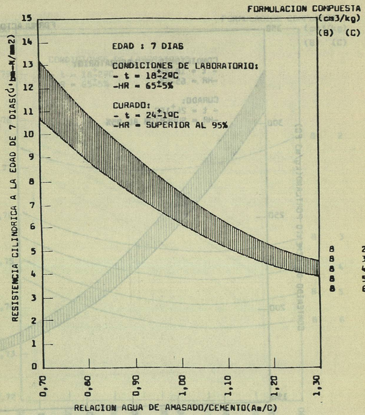
FIG. 5 - HORMIGON CELULAR SUPERPLASTICO (Ac=20±2cm) RESISTENCIA CILINDRICA A LA EDAD DE 7 DIAS (kg/cm 2 ), EN FUNCION DE LA RELACION AGUA DE AMASADO/CEMENTO (Aa/C), Y DE LA FORMULACION COMPUESTA EMPLEADA (POR INTERPRETACION DE VALORES MEDIOS EXPERIMENTALES).
