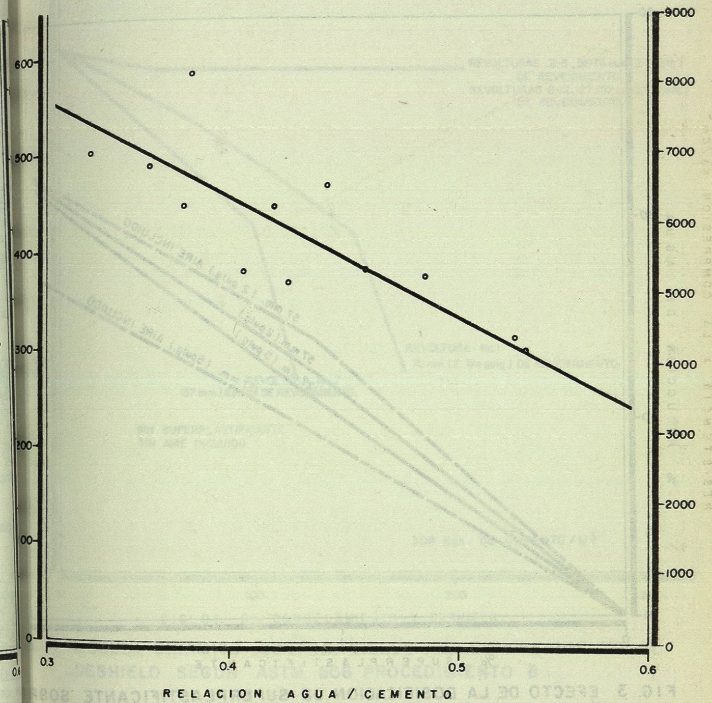
2 RELACION DE RESISTENCIA A LA COMPRESION PARA CONCRETO CON AIRE INCLUIDO Y CON SUPERPLASTIFICANTE - CONTRA RELACION AGUA / CEMENTO.
