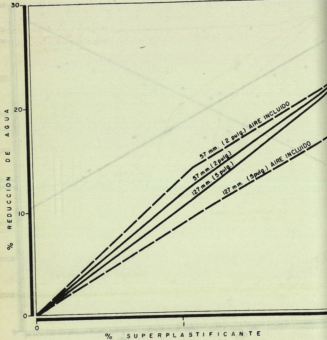
FIG. 3 EFECTO DE LA DOSIFICACION DE SUPERPLASTIFICANTE SOBRE LA REDUCCION DE AGUA.
