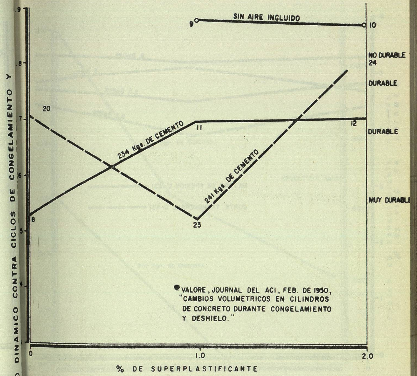
FIG. 5 MODULO DINAMICO CONTRA CICLOS DE CONGELAMIENTO Y DESHIELO. COEFICIENTE DE SATURACION CONTRA DOSIFICACION DE SUPERPLASTIFICANTE PARA CONCRETO CON AIRE INCLUIDO.
