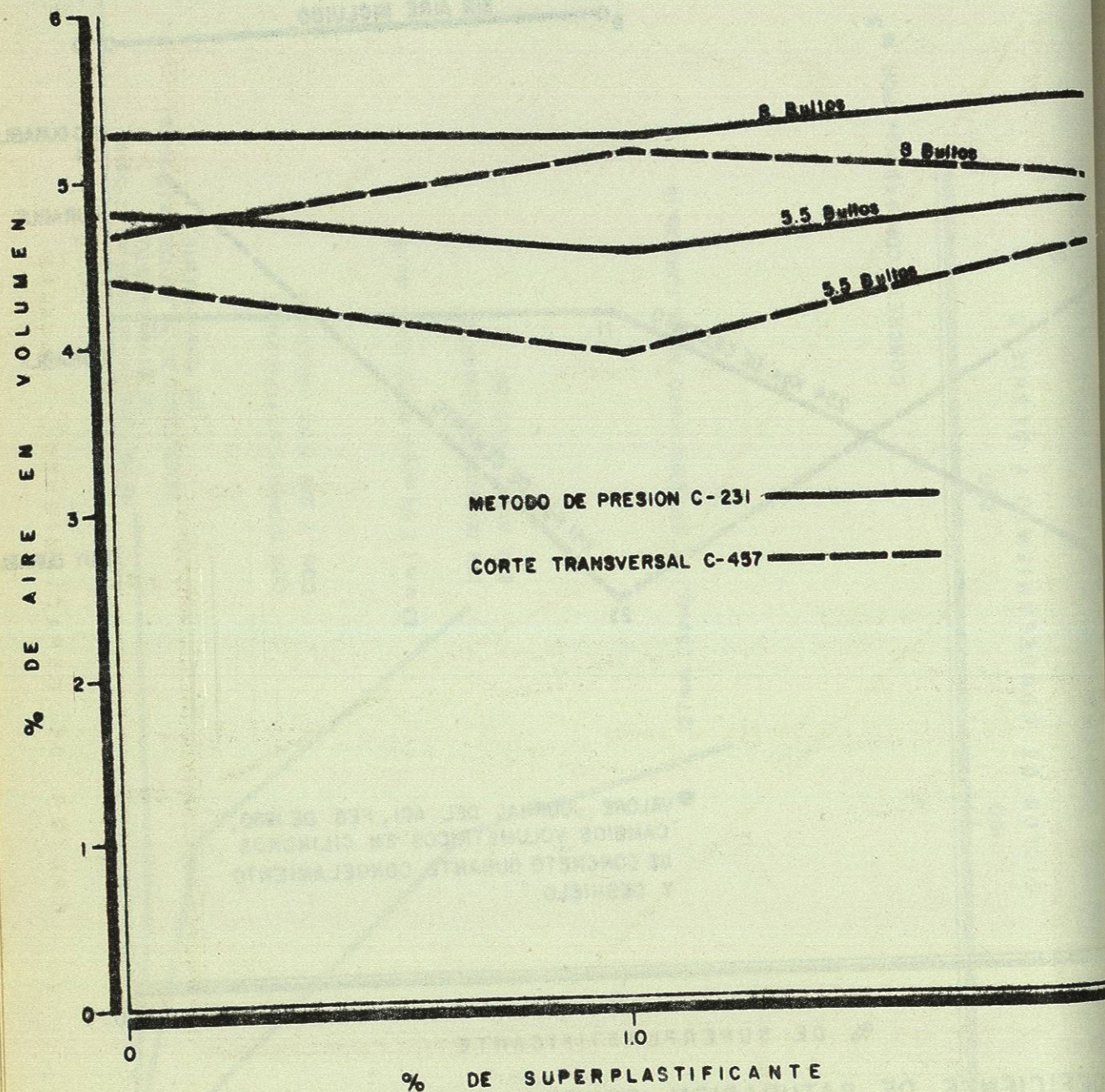
FIG. 7 COMPARACION ENTRE EL CONTENIDO DE AIRE EN CONCRETO FRESCO (METODO DE PRESION C-231) Y CONTENIDO DE AIRE EN CONCRETO ENDURECIDO C-457.
