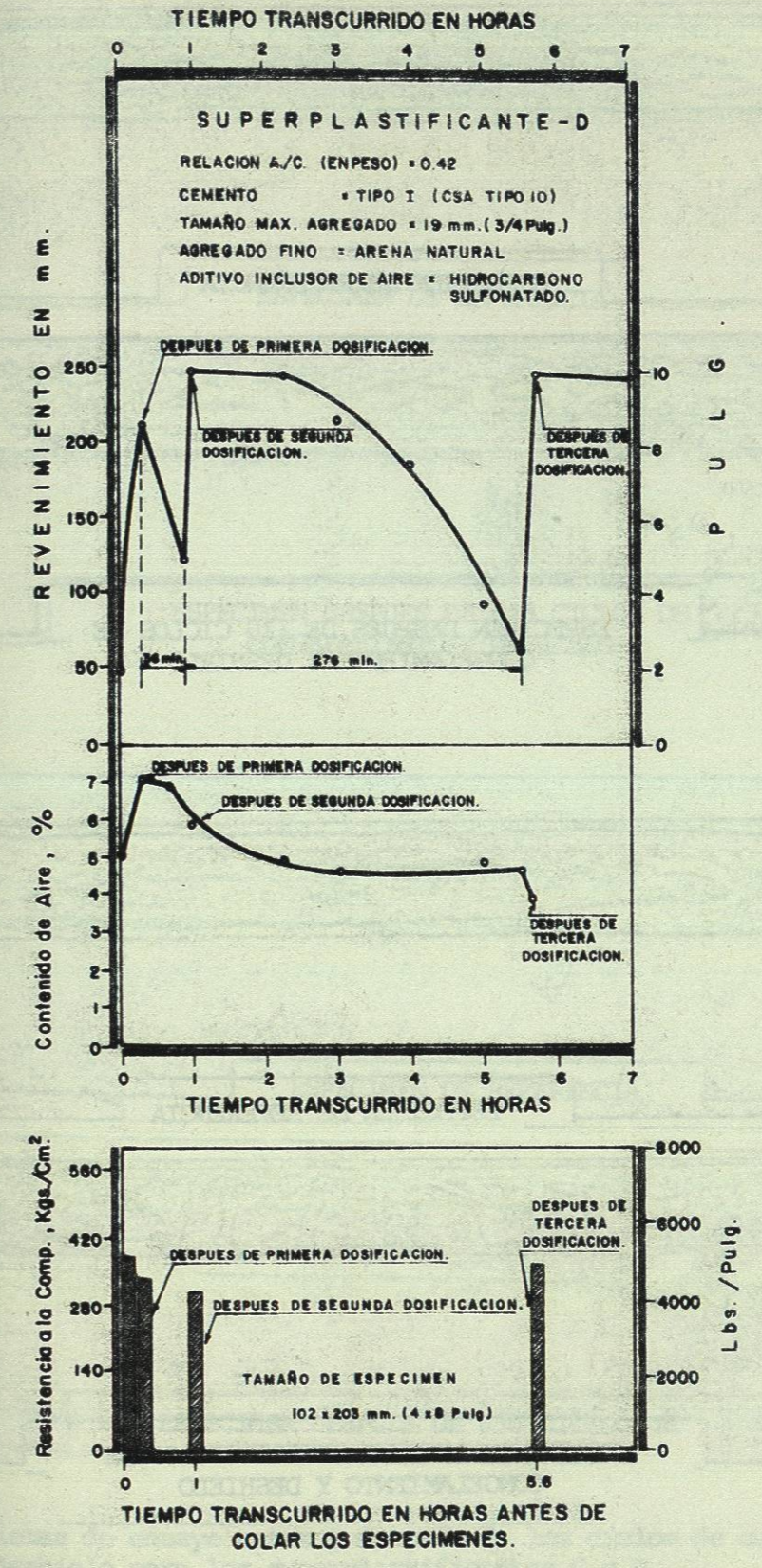
FIG. 5 TIEMPO TRANSCURRIDO DESDE EL MEZCLADO INICIAL CONTRA REVENIMIENTO, CONTENIDO DE AIRE Y RESISTENCIA A LA COMPRESION SUPERPLASTIFICANTE - D.
