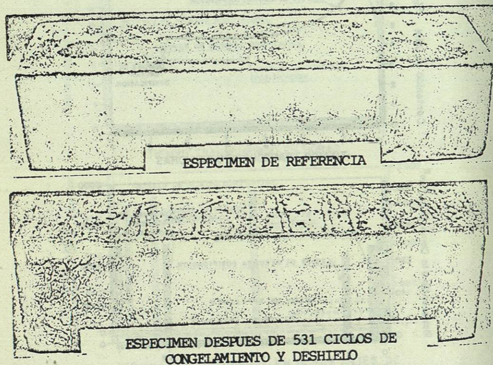
Fig. 6.- Prismas de ensaye antes y después de los ciclos de congelamiento y deshielo para los superplastificantes A y B.
