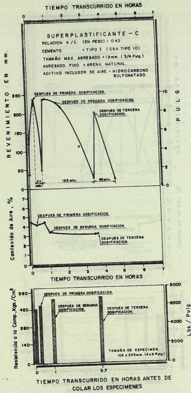
FIG. 4 TIEMPO TRANSCURRIDO DESDE EL MEZCLADO INICIAL CONTRA REVENIMIENTO, CONTENIDO DE AIRE Y RESISTENCIA A LA COMPRESION SUPERPLASTIFICANTE - C.
