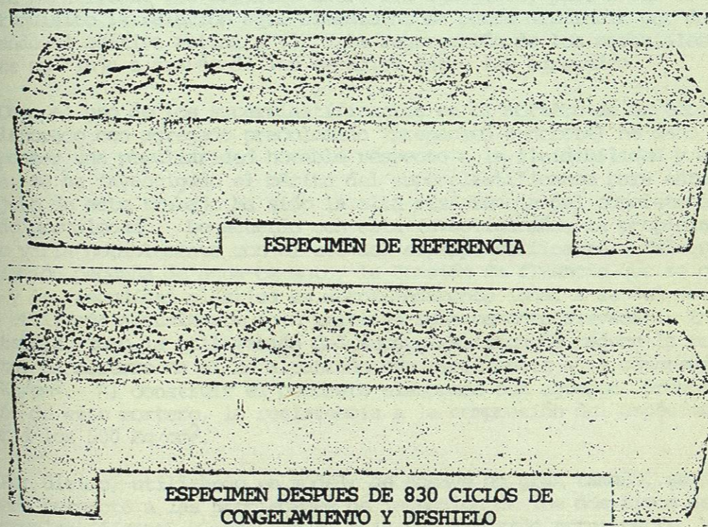
Fig. 7.- Prismas de ensaye antes y después de los ciclos de congelamiento y deshielo para los superplastificantes C y D.
