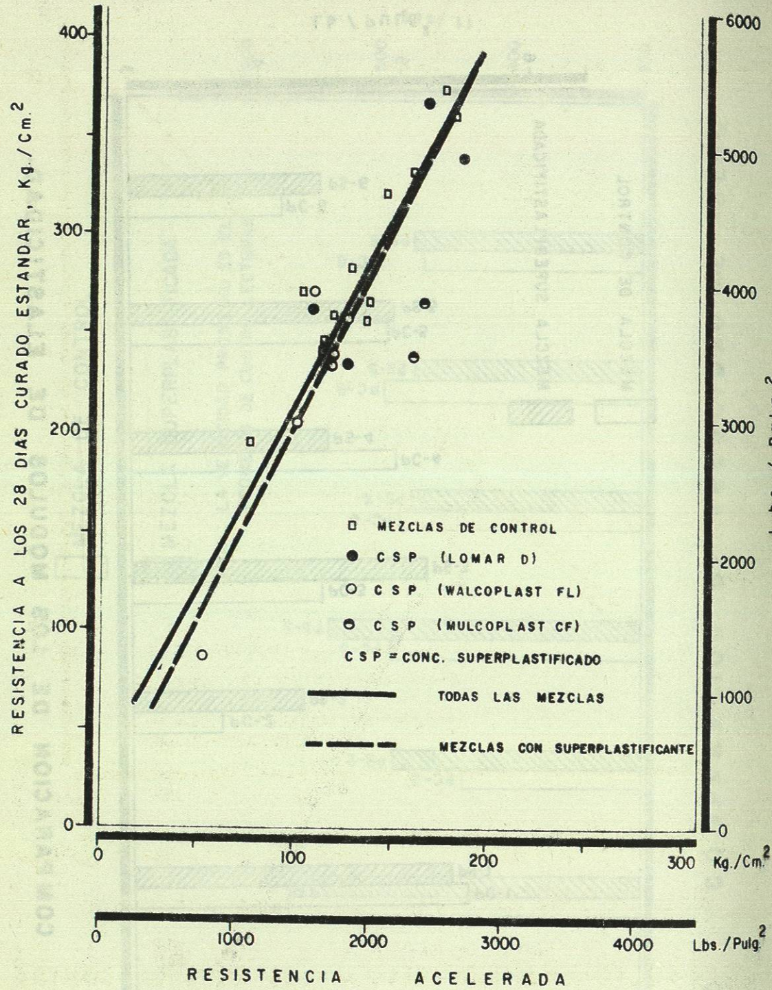
FIG. 12 RESISTENCIA A LOS 28 DIAS VS. RESISTENCIA ACCELERADA.
