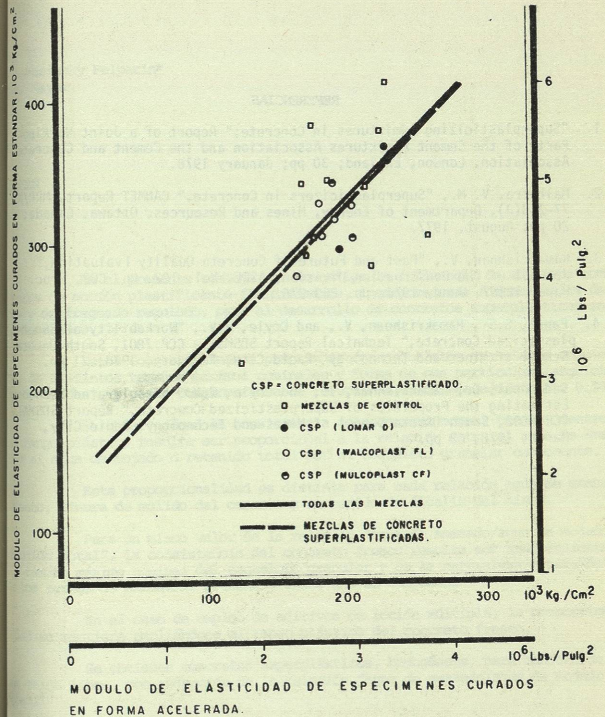
FIG.15 MODULO DE ELASTICIDAD DE ESPECIMENES CURADOS EN FORMA ACCELERADA VS. MODULO DE ELASTICIDAD DE ESPECIMENES CURADOS EN FORMA ESTANDAR.
