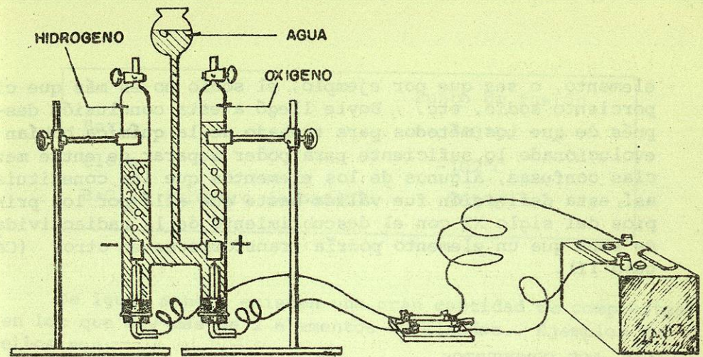
Fig. 1-1. Electrólisis del agua.
