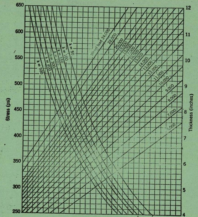
Gráfica de Diseño para pavimentos rígidos. Método de la P. C. A.
