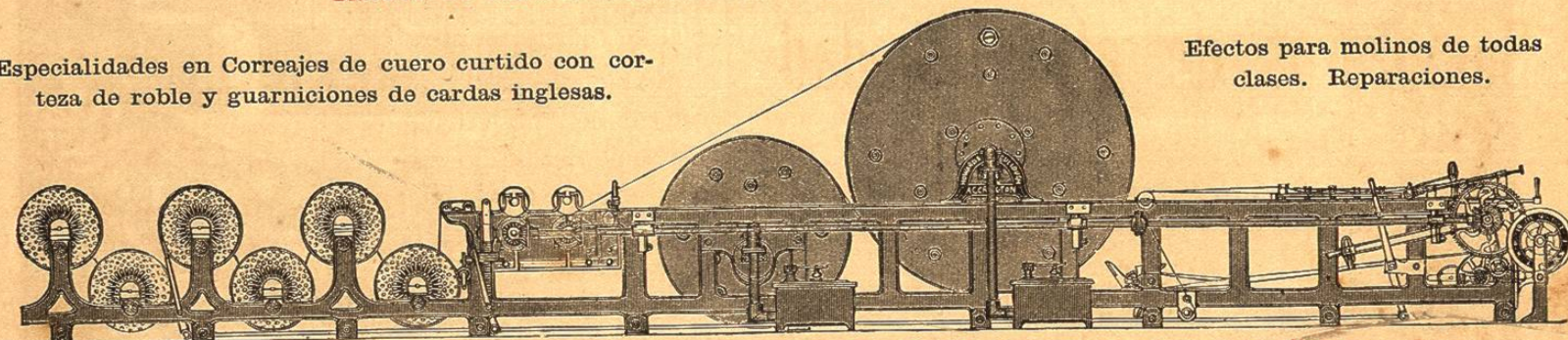
CALANDRIAS PERFECCIONADAS DE PATENTE, MAS DE 800 EN OPERACION SOLO EN AMERICA.
