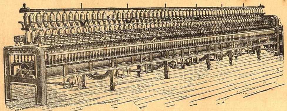
BANCOS DE HILAR PERFECCIONADOS. 1,200,000 CANILLAS EN OPERACION.
