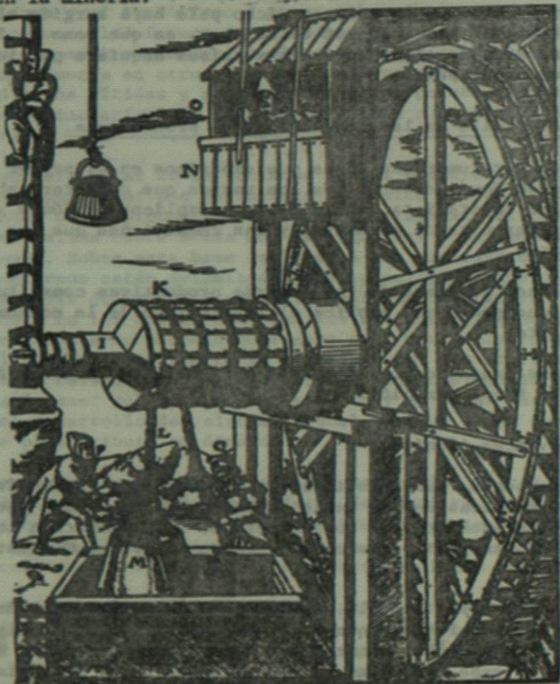
Rueda de arcaduccs para extraer el agua de las minas. Agrícola, 1556.
