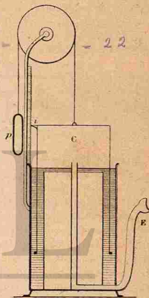
Fig. 43. Schéma du spiromètre. (D'après L. Frédéricq; Manipulations de Physiologie .) C, cloche graduée. — p, contre poids. i, index. — E, embouchure.
