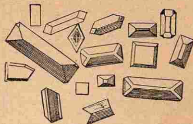
Fig. 54. — Phosphate ammoniaco-magnésien.
