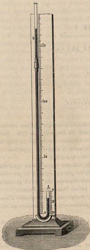
Fig. 120. — Tube de Mariotte.
