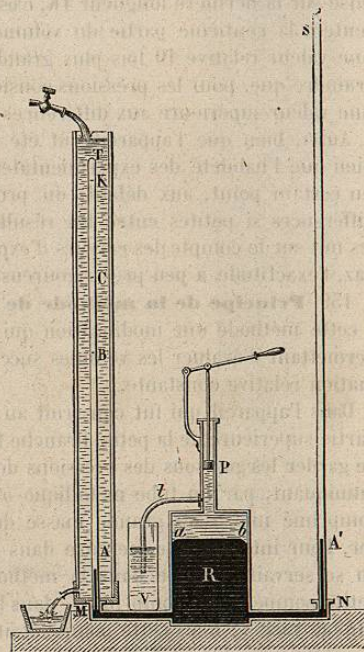
Fig. 128. — Appareil de Dulong et Arago.
