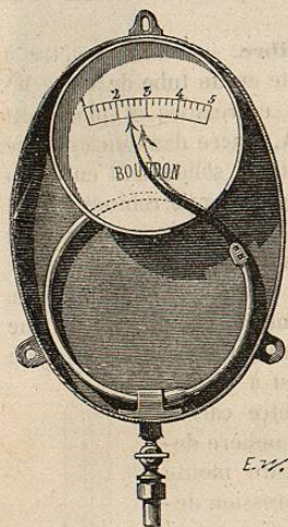
Fig. 133. — Manomètre métallique.
