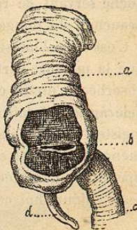
Fig. 52. — Valvule éo-cæcale (*).
