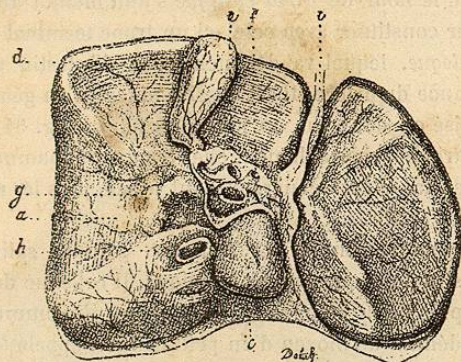
Fig. 54. — Foie (*).
