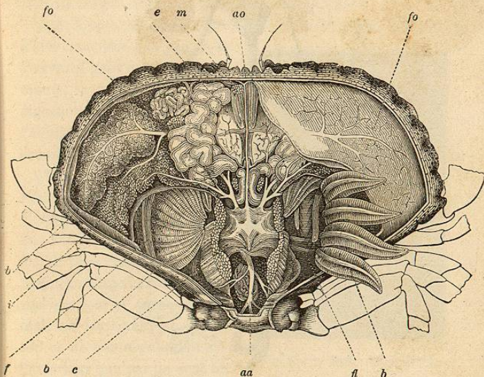
Fig. 56. — Anatomie d'un Crabe tourteau (*).
