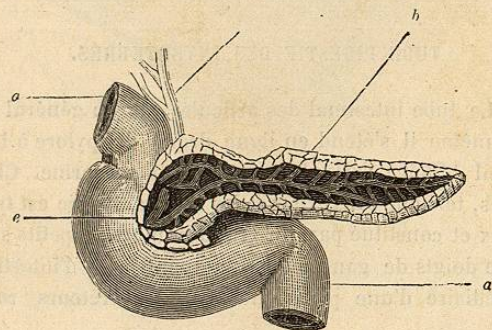
Fig. 55. — Pancréas (**).
