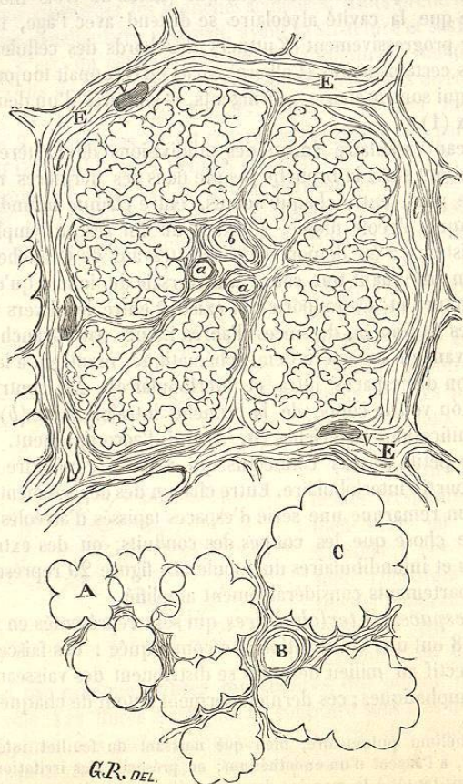
FIG. 28 et 29. — Coupe transversale du lobule pulmonaire (J. Grancher). — a. ramification de l'artère pulmonaire; b. bronche intra-lobulaire; E. espaces lobulaires; V. veines; L. espaces lymphatiques.
