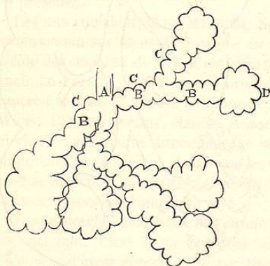
FIG. 27. — Coupe de l' acinus pulmonaire.
