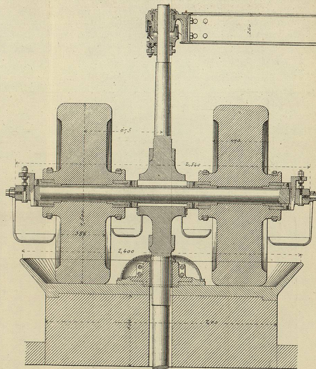
Fig 5 Elévation - coupe.
