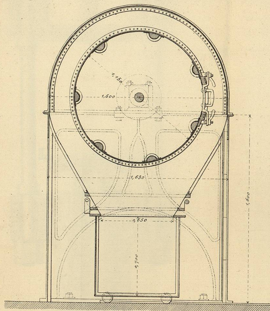
Fig 1. Elévation - coupe transversale.
