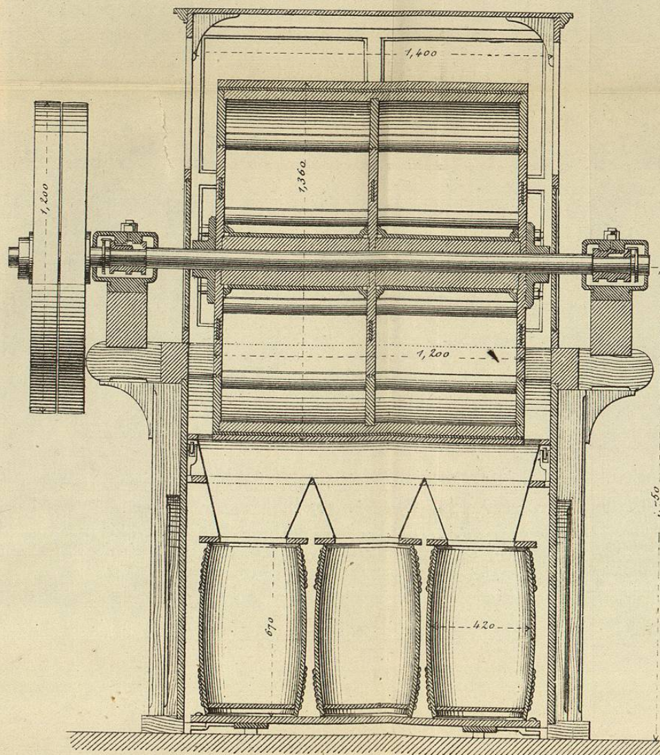
Fig 4. Elévation - coupe longitudinale.
