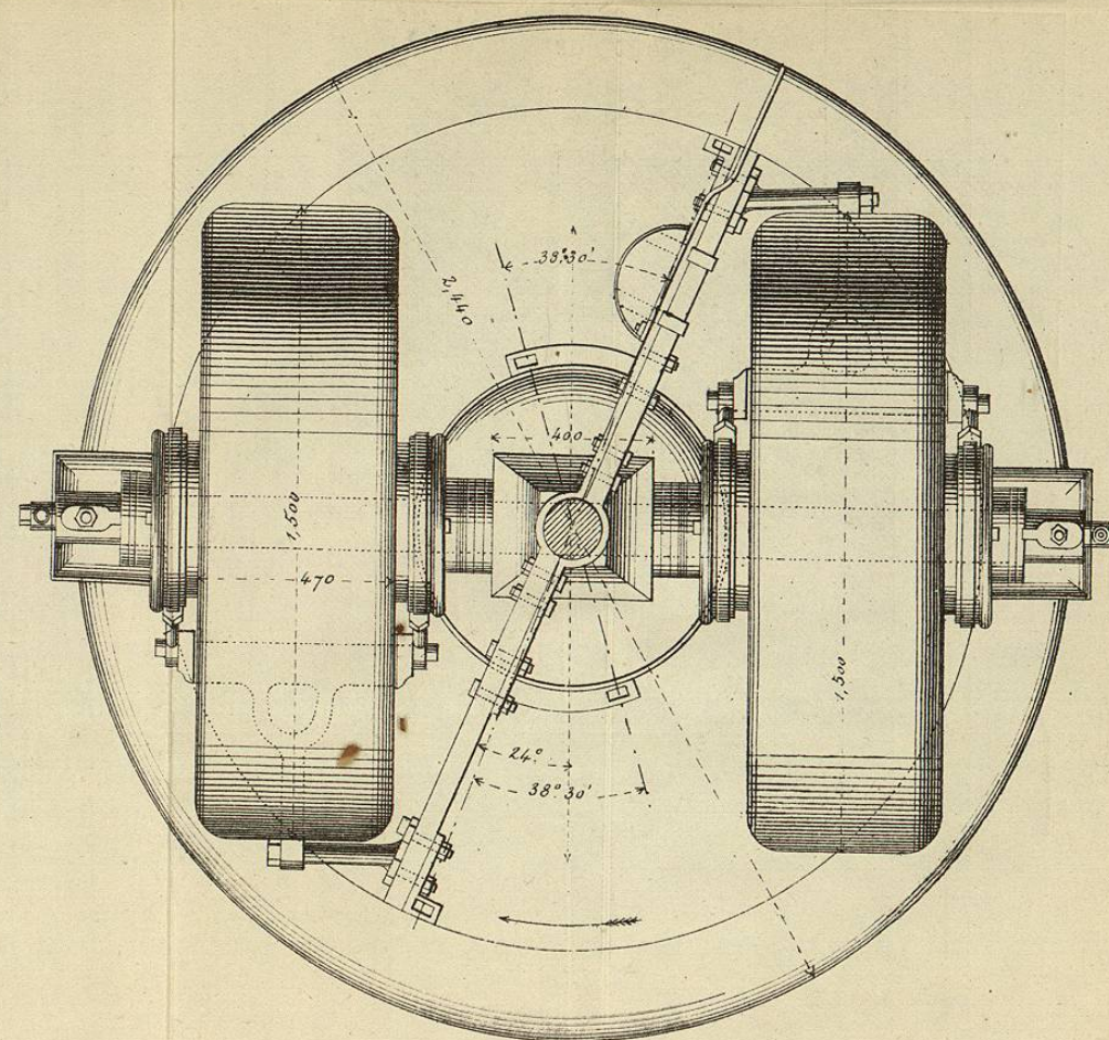
Fig 6. Plan - coupe.
