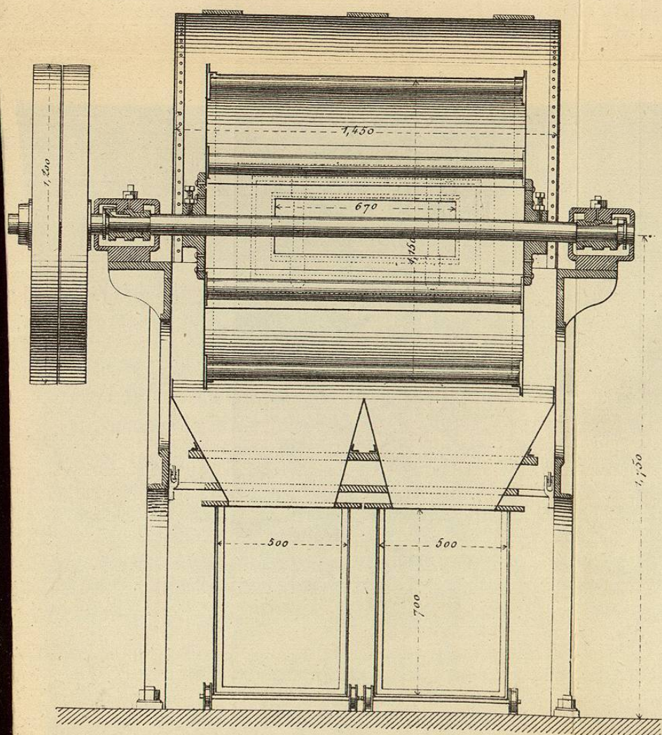
Fig 2. Elévation - coupe longitudinale.
