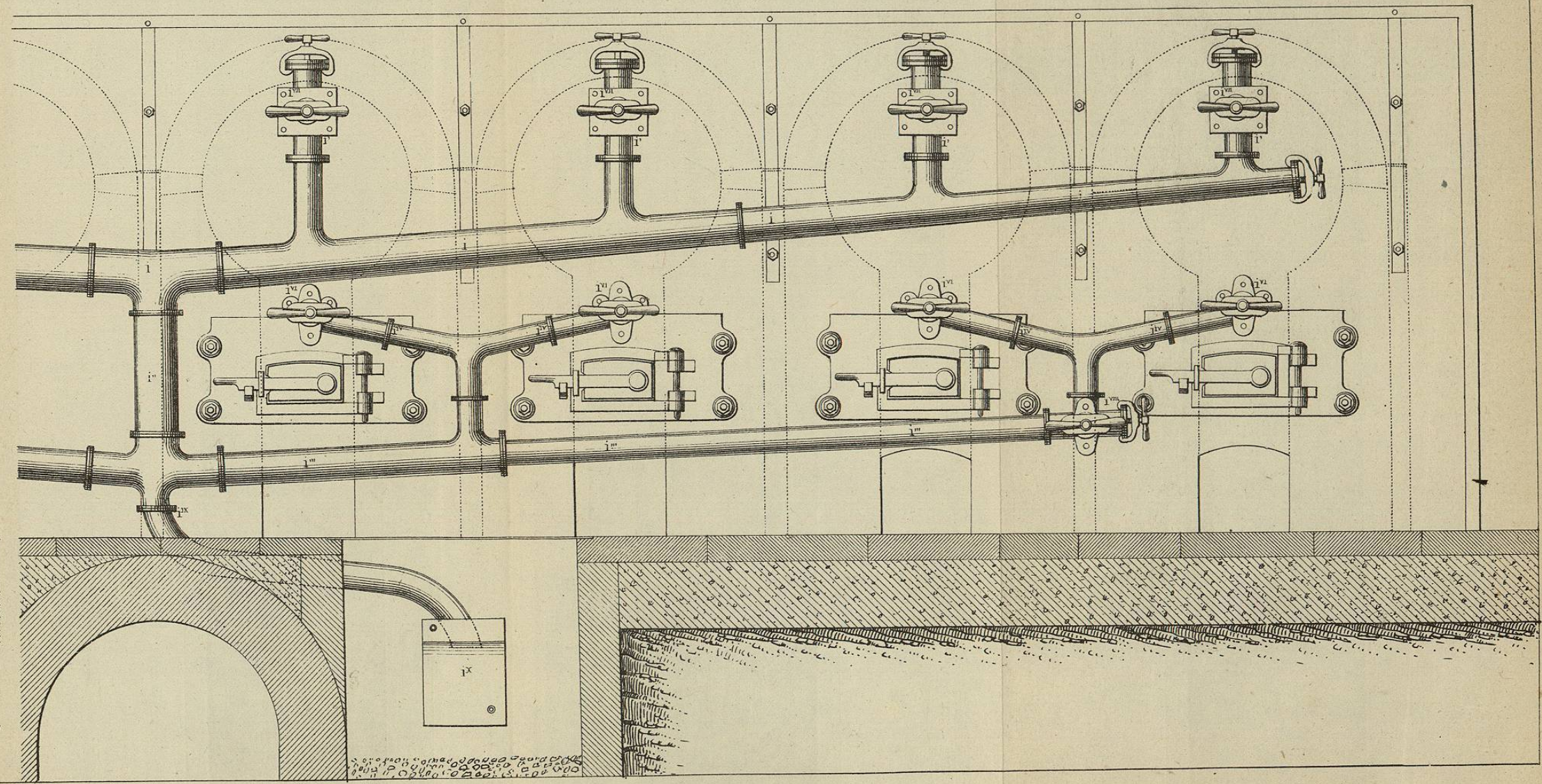
Fig.2. Elévation postérieure.
