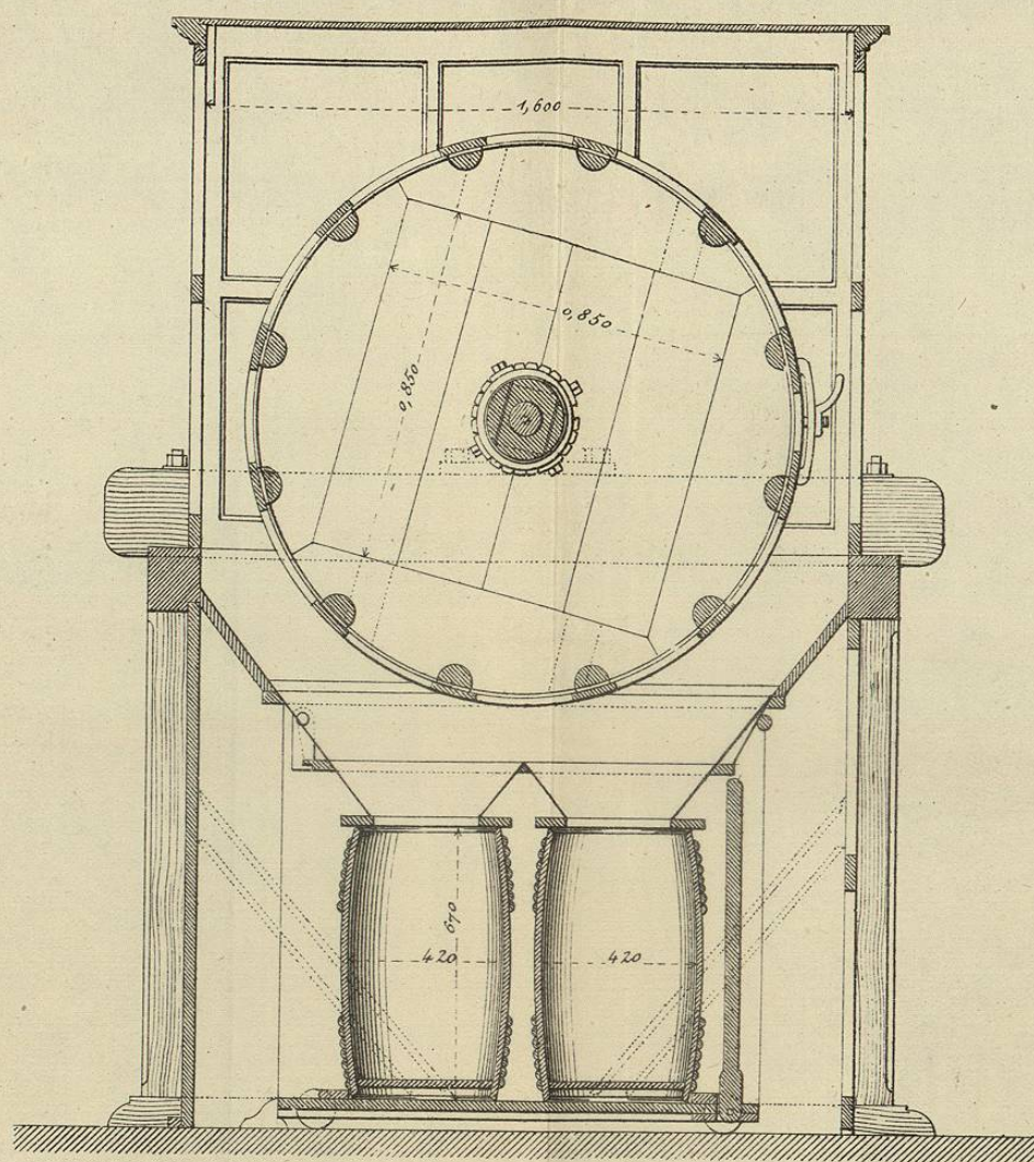
Fig 3. Elévation - coupe transversale.
