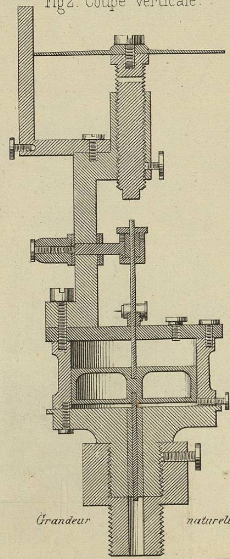
Fig 2. Coupe verticale.
