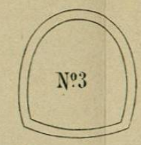
Forma que correspondiera dar a la sección transversal de un socabón de bóveda.
