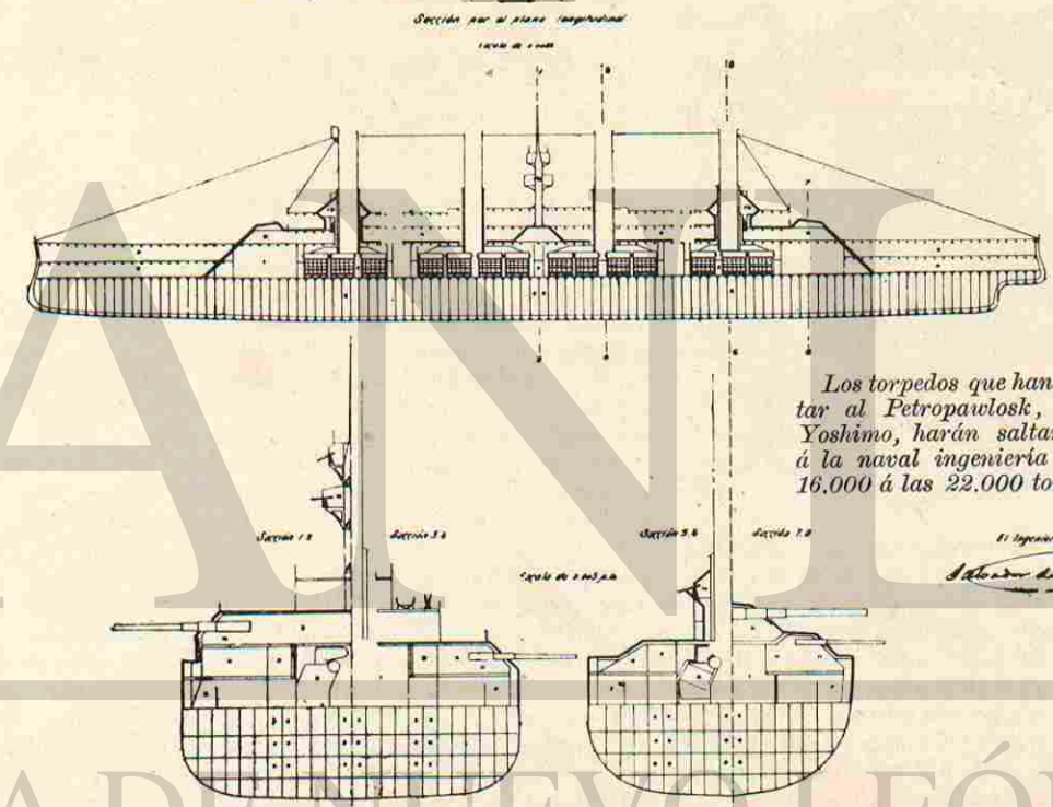
Buque de combate invulnerable á la Artillería y los Torpedos
