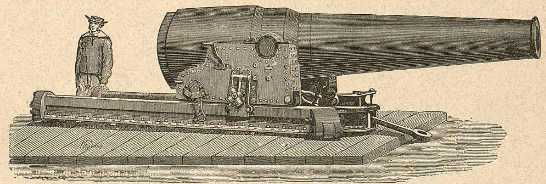
CAÑON DE 0.24 Y CUREÑA
