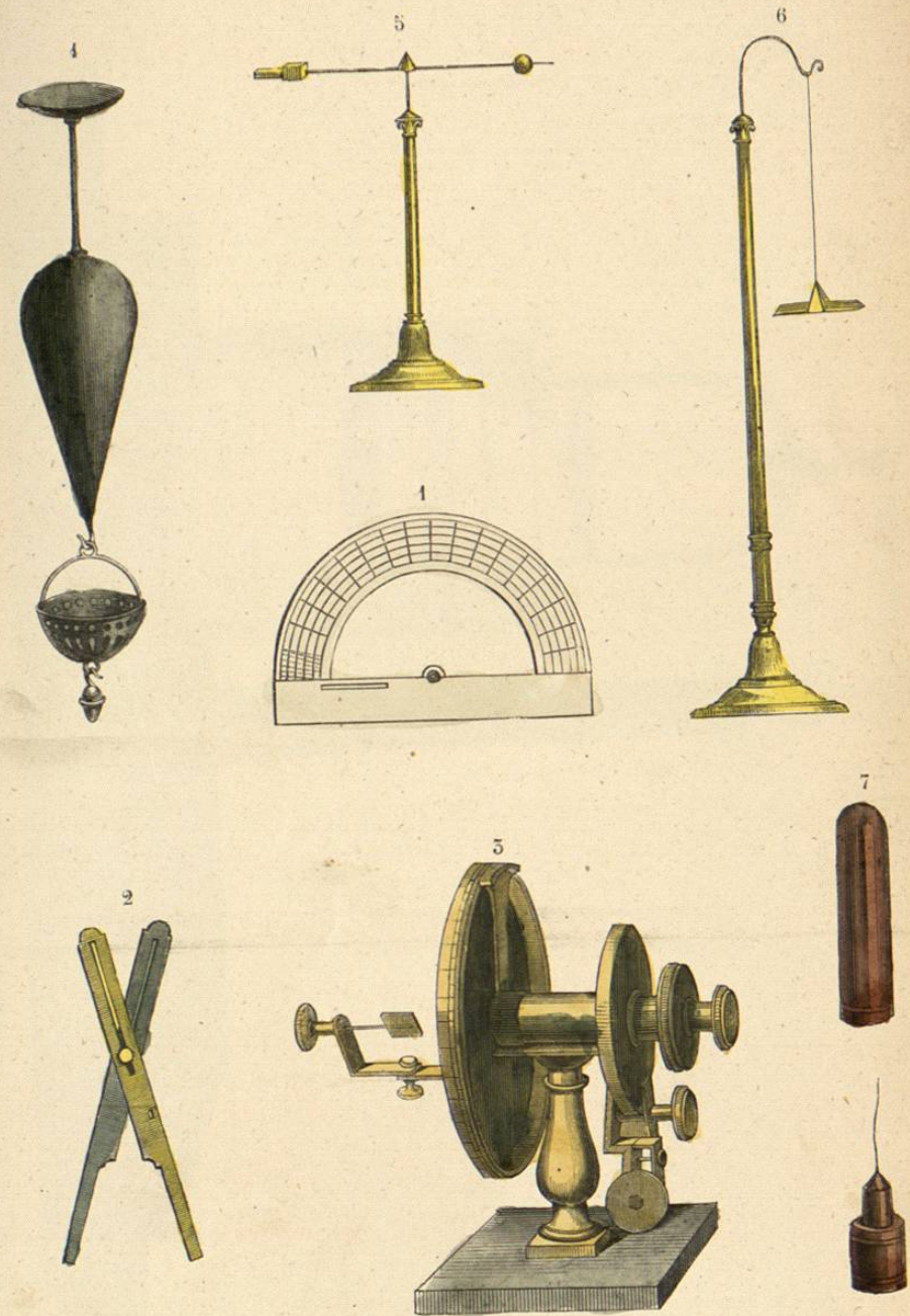
1 y 2. Compás y semicírculo graduado del goniómetro de aplicación.—3. Goniómetro de Wollaston.—4. Gravímetro ó balanza de Nicholson.—5. Electrómetro de Haüy.—6. Sostén de Turmalina.—7. Electróscopo de pelo de gato.
