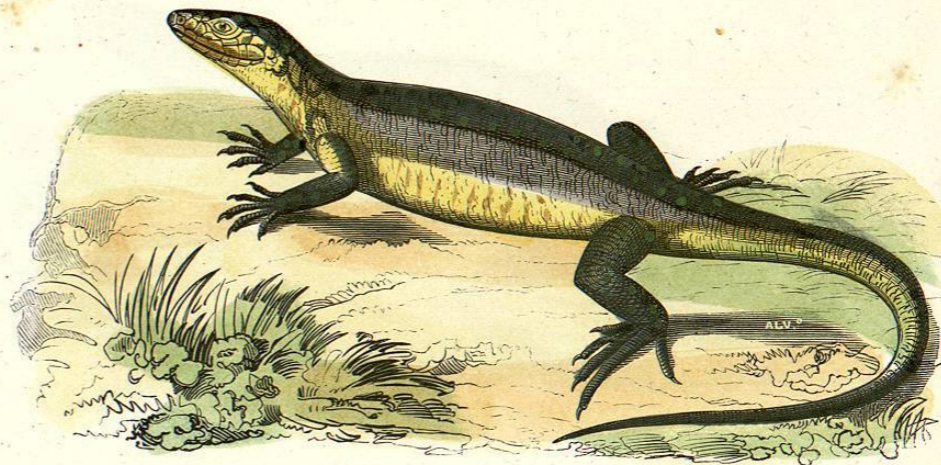
SCINCUS DUMERILII.
