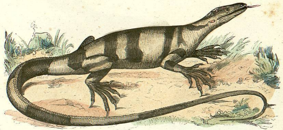
VARANUS BELLII.
