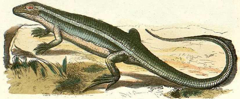
GHERROSAURUS BIFASCIATUS.
