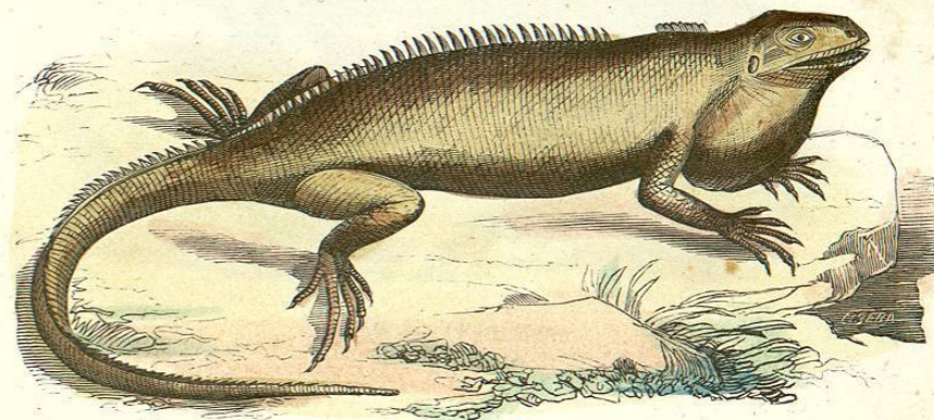
ALOPNOTUS RICORDII.
