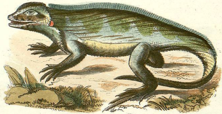
HOLOTROPIS HERMINIERI.
