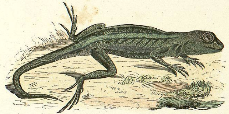
TROPIDOGASTER BLAINVILLII.
