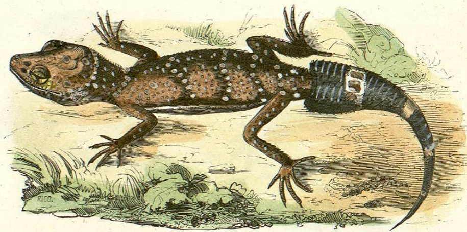
GYMNODACTYLUS MILIUSII.
