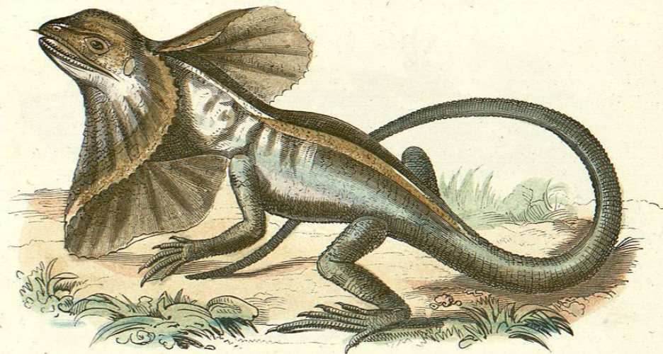
CHLAMYDOSAURUS KINGII.
