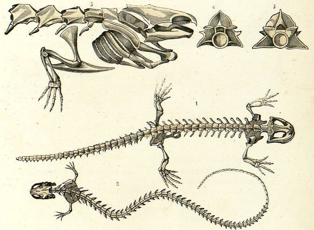
1. Salamandra vulgaris.
