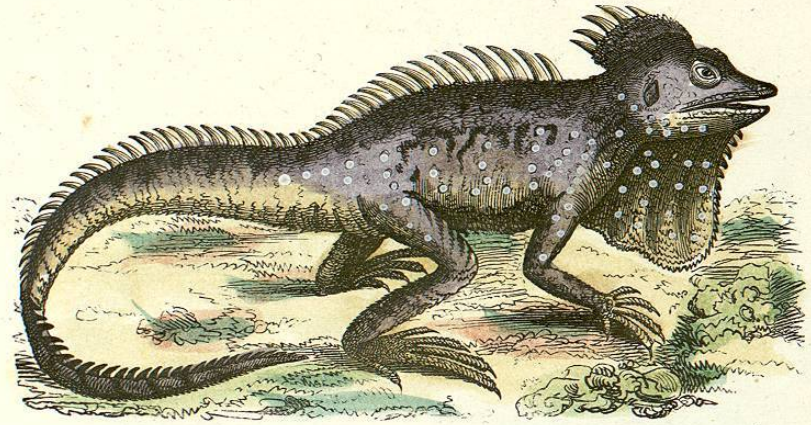
TIARIS DILOPHUS.
