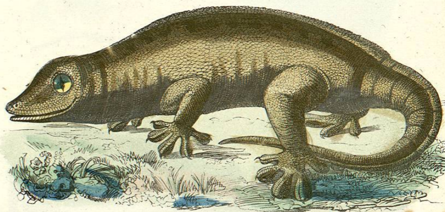
PLATYDACTYLUS SEYCHELLENSIS.
