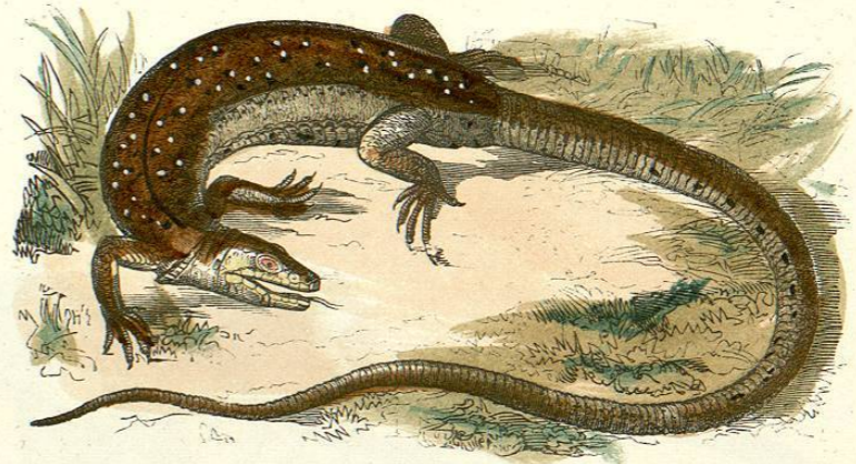
LACERTA DELALANDII.
