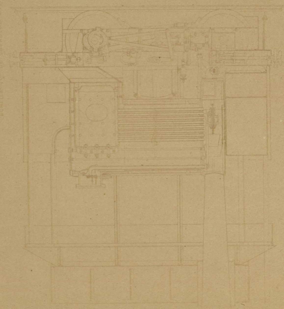
ТУРБЕНА ДЕ АДИЕ 1200 ЦИЛИНДЕР 0 м 125. ДИАМЕТР ЦИЛИНДРА 0 м 61. КОМПАНИЈА ДЕ ЛУВМУА ДЕ И. И. МЕРКАТУИМЕР & ФИЛС
