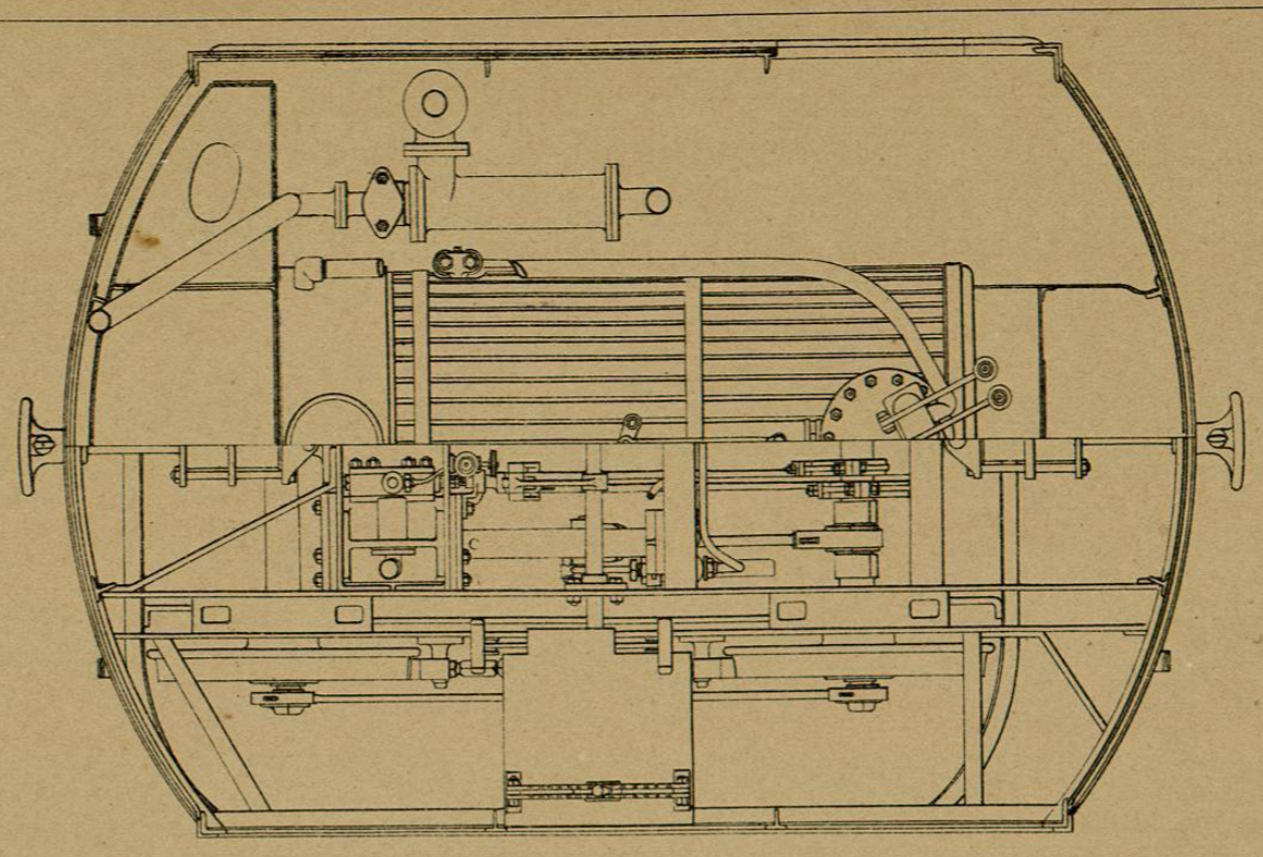
CYLINDRES 0 м 152 x 0 м 228. DIAMETRE DES ROUES 0 м 61. LARGEUR DE VOIE 1 м 00.
