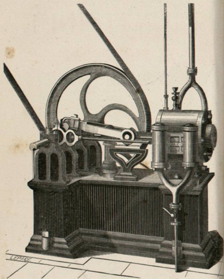
LE MOTEUR A GAZ.
