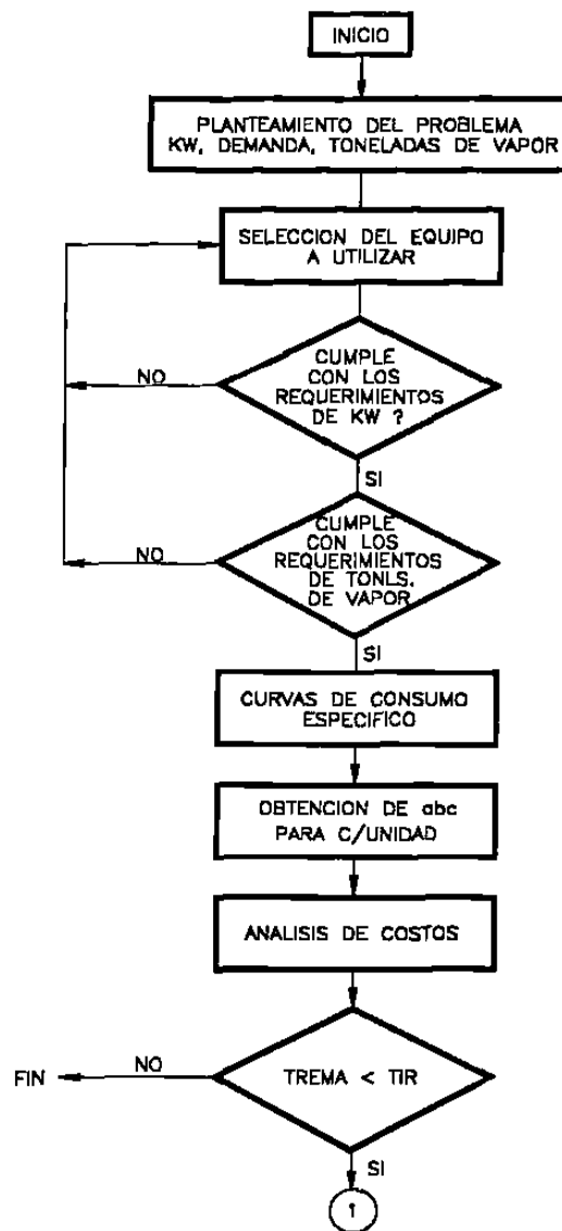
DIAGRAMA DE FLUJO PARA LA METODOLOGIA PROPUESTA
