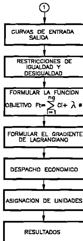
DIAGRAMA DE FLUJO PARA LA METODOLOGIA PROPUESTA Fig. #12(Continuación).
