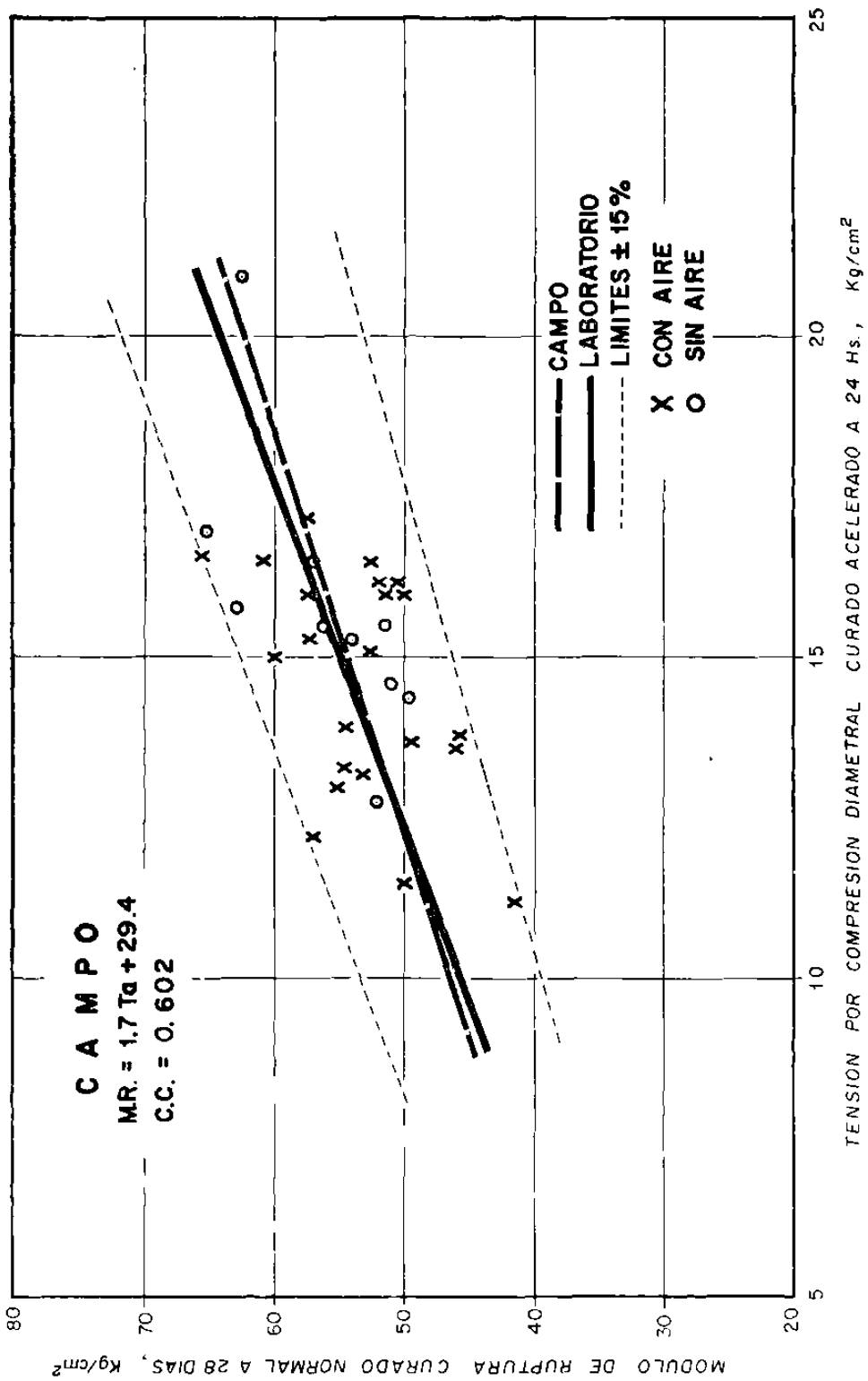
FIG.17 RELACION ENTRE LA TENSION C.D. ACEL. A 24 Hs. Y EL M.R. NORMAL A 28 DIAS.
