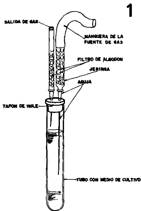
FIG. 1.- APARATO UTILIZADO PARA GASEAR LOS CULTIVOS CON CO 2 .
