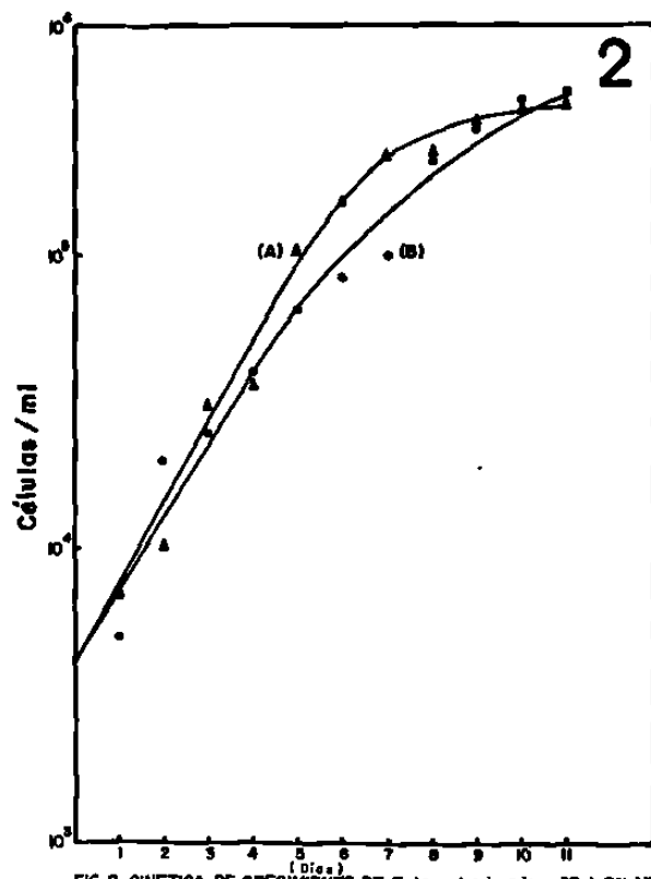
FIG. 2.- CINÉTICA DE CRECIMIENTO DE Entamoeba invadens IP-1 EN MEDIO TP-S-1. CURVA A (▲) CON TENSIÓN NORMAL DE CO 2 , CURVA B (●) CON ALTA TENSIÓN DE CO 2 .
