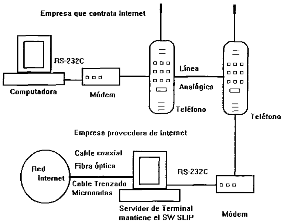
Figura 4.2 Conexión Conmutada
