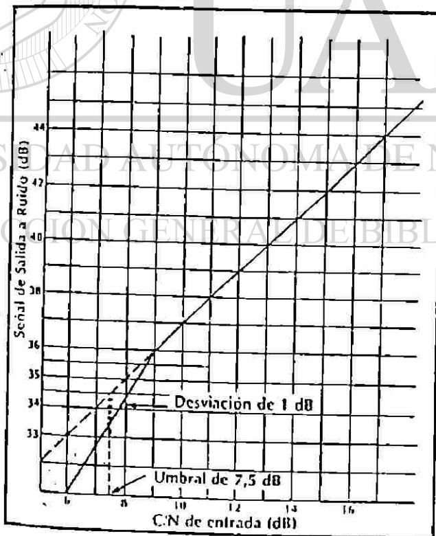
2-43. Umbral del Receptor. Una estación terrestre debería proporcionar una razón C/N lo suficientemente alta como para exceder el umbral del receptor. El umbral se mide en el punto donde la desviación de la linealidad es de 1 decibel.
