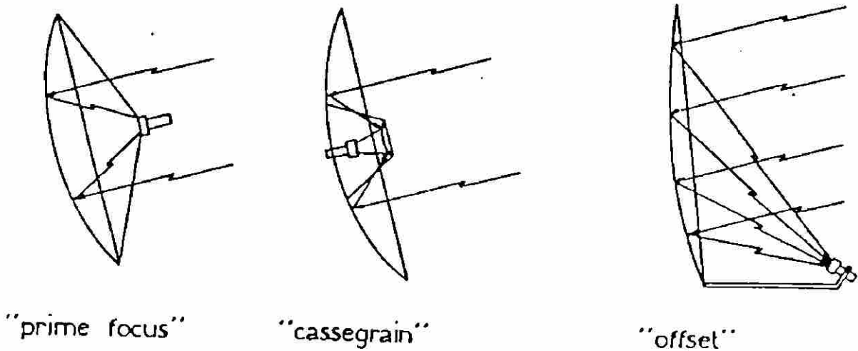
Los principales tipos de alimentación en la configuración de las parábolas: tipo foco primario, offset y Cassegrain
