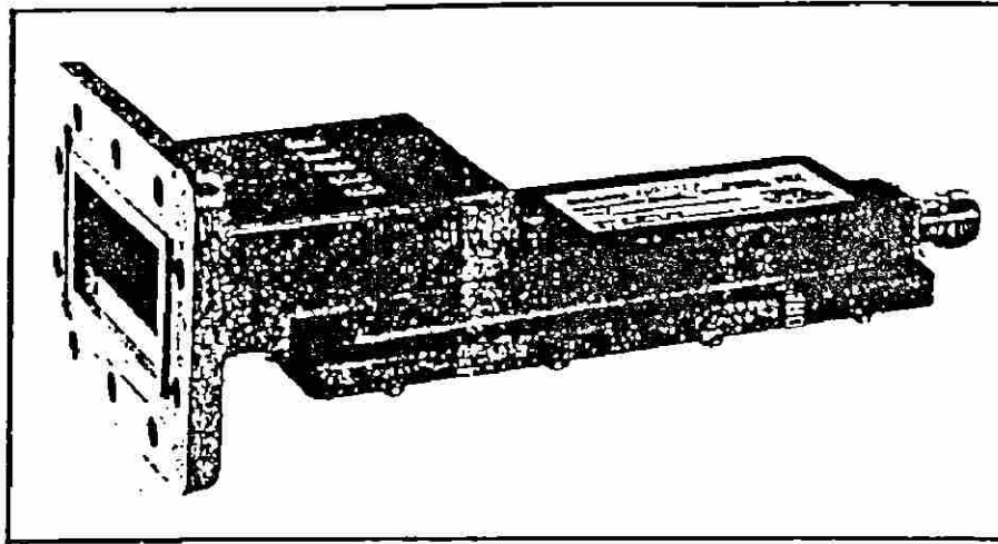
LNA Drake. Hay fabricantes, como la compañía R.L. Drake, que ofrecen los LNA con una gama de diferentes temperaturas de ruido. (Cortesía de la R.L. Drake Company).
