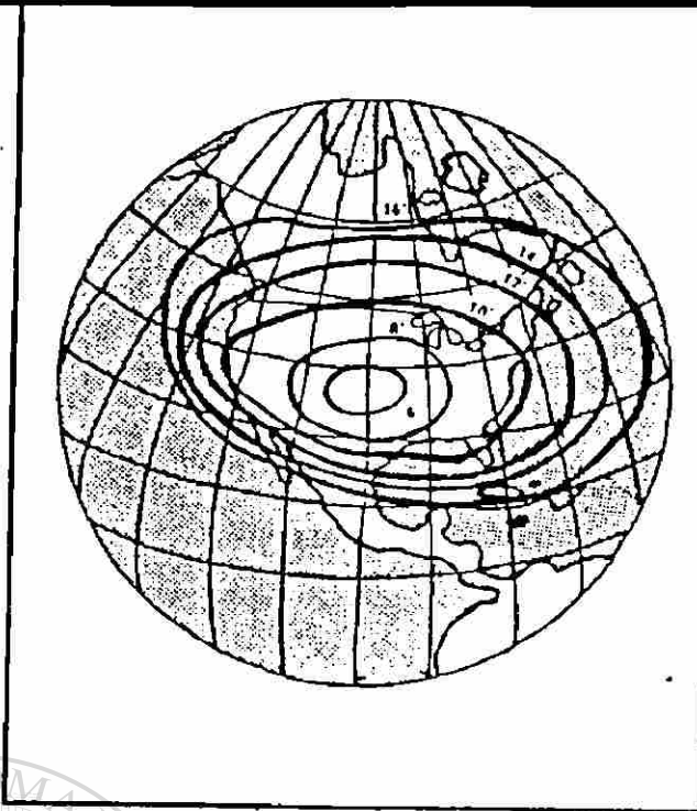
Mapa de Pisada y Tamaño de la Antena. Muchos mapas de pisada, en lugar de mostrar los contornos EIRP, muestran el diámetro mínimo de antena requerido.
