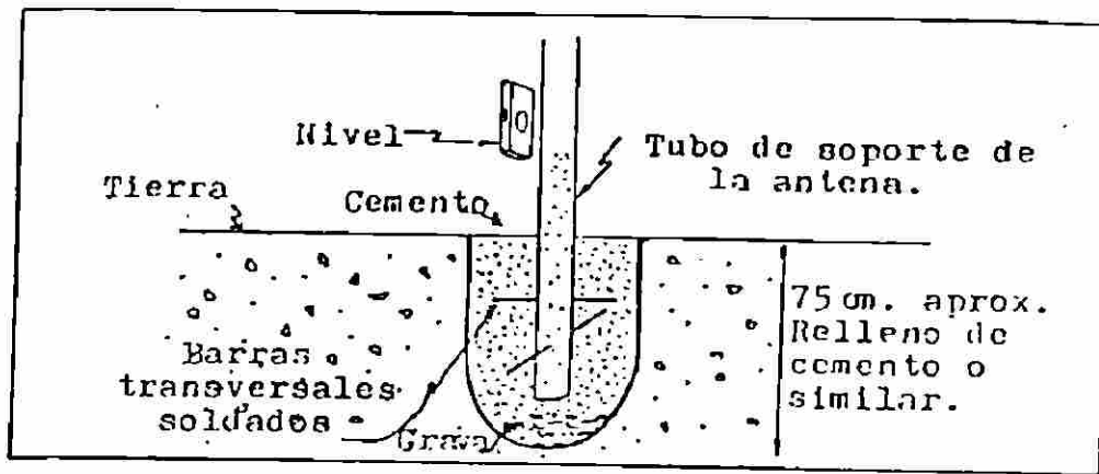
TIPOICO SOPORTE DE POSTE DE ANTENA
