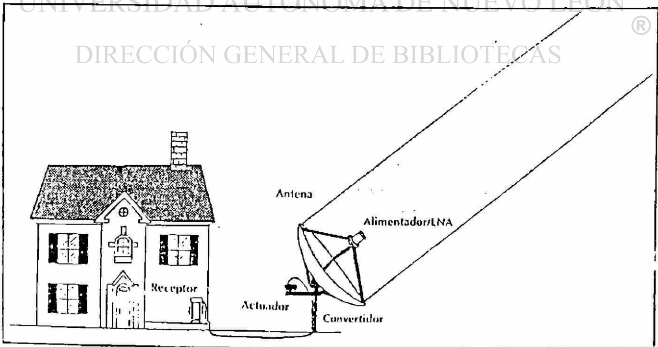
Estación Terrestre Típica. Las señales captadas por la antena son enfocadas hacia el alimentador y el amplificador de ruidos bajos. Luego son transmitidas por cable hacia el convertidor, y de ahí a un receptor de satélite modulador. El sistema puede alimentar cualquier número de equipos de televisión.
