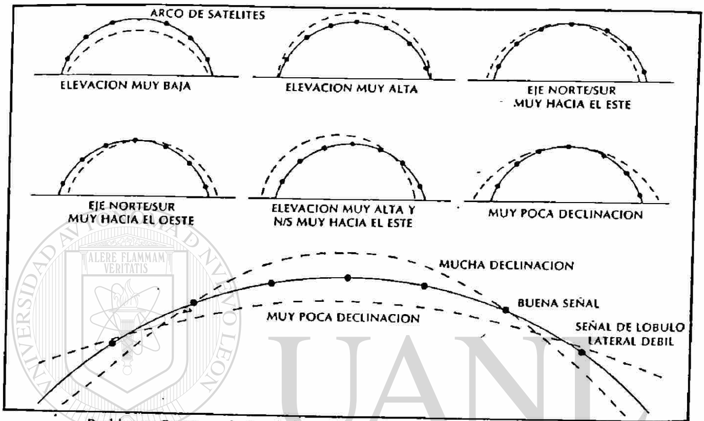
Problemas Comunes de Seguimiento de Antena. Casi todos estos problemas se deben a una orientación nort/sur incorrecta. Sin embargo, si no se ha ajustado bien el ángulo de declinación, tampoco habrá un buen seguimiento. Para alinear la antena con el arco geosíncrono de los satélites basta alinear dos semicírculos, el de los satélites con el que traza el soporte polar.
