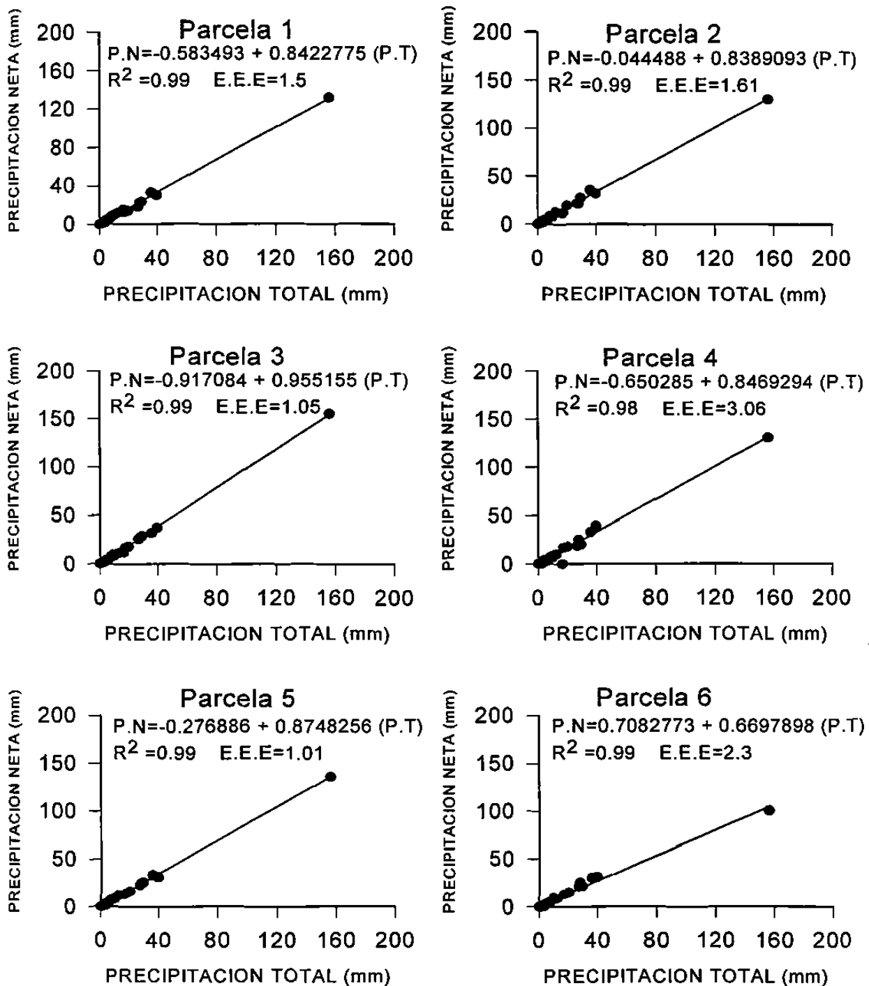
Figura 3. Relación entre la precipitación neta y la precipitación total para seis parcelas de una comunidad semi-árida del nordeste de México.
