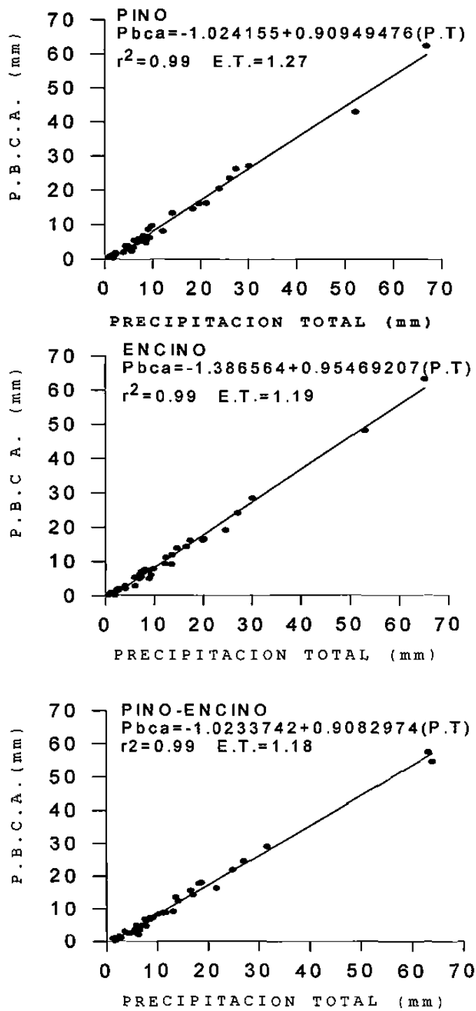
Figura 11. Relación entre la precipitación bajo la cobertura arbustiva y la precipitación total en tres tipos de bosques del nordeste de México.
