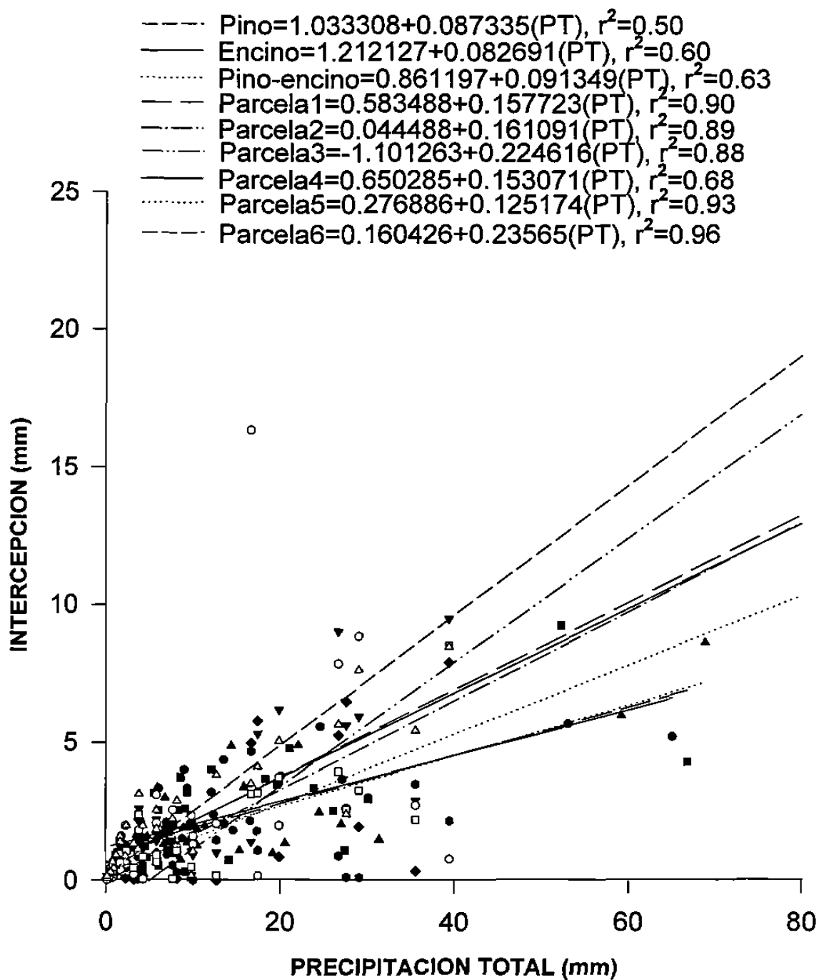
Figura 18. Relación entre la intercepción y la precipitación total entre los rodales de pino, encino, pino-encino y las seis parcelas del matorral espinoso tamaulipeco
