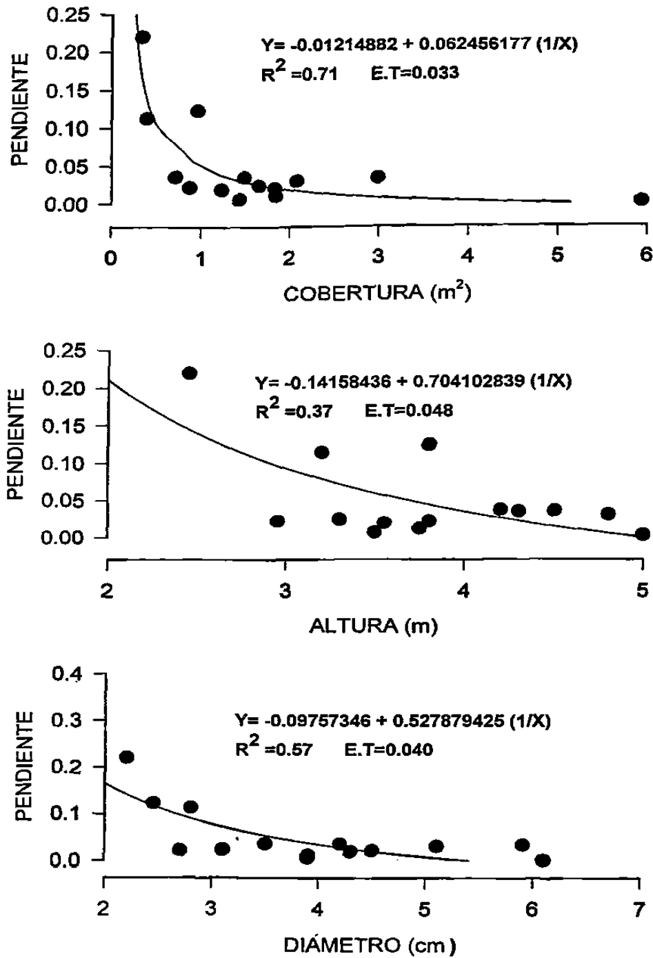
Figura 8. Relación entre la pendiente del escurrimiento fustal y 3 características dasométricas de los arbustos de A. rigidula .
