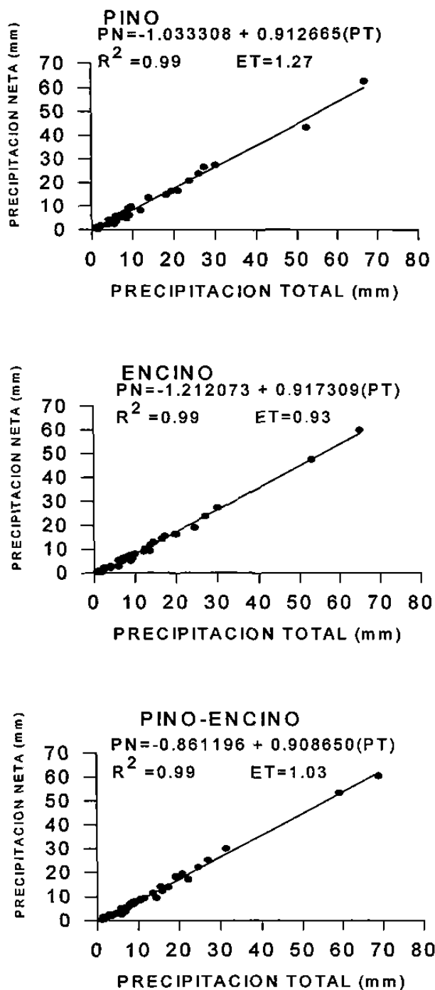
Figura 10. Relación entre la precipitación neta y la precipitación total en tres tipos de bosques del nordeste de México.
