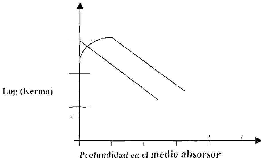
Gráfica 1.- Relación entre el Kerma y la dosis para radiación de fotones
