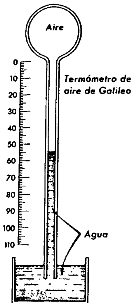
Fig. 27 A. El aire al calentarse se expande y empuja al agua hacia abajo en el tubo. Al enfriarse, el aire se contrae y el agua sube.
