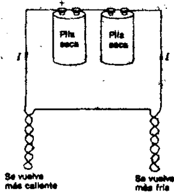
Fig. 36-9 Efecto Peltier.
