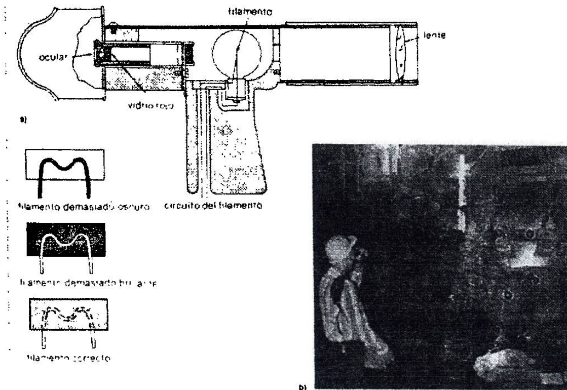
Figura 168.3 Pirómetro óptico. a) El filamento permite hacer una comparación visual de brillos que se iguala a un "trasfondo" de temperatura. La corriente que pasa por el filamento es proporcional a la temperatura. b) Un pirómetro óptico que se usa para medir la temperatura de acero fundido.
