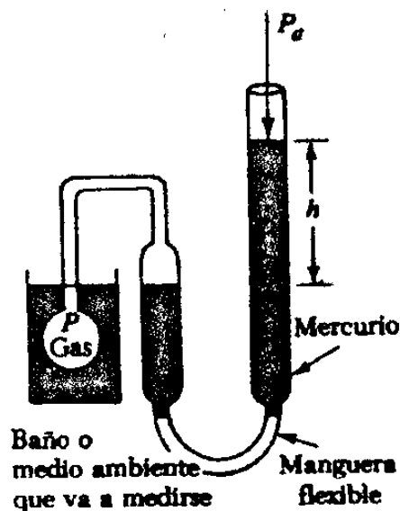
Fig. 16.2 Un termómetro de gas a volumen constante mide la presión del gas contenido en la botella de la izquierda. El volumen del gas en la botella se mantiene constante elevando o bajando la columna de la derecha, de tal forma que el nivel del mercurio permanezca constante.
