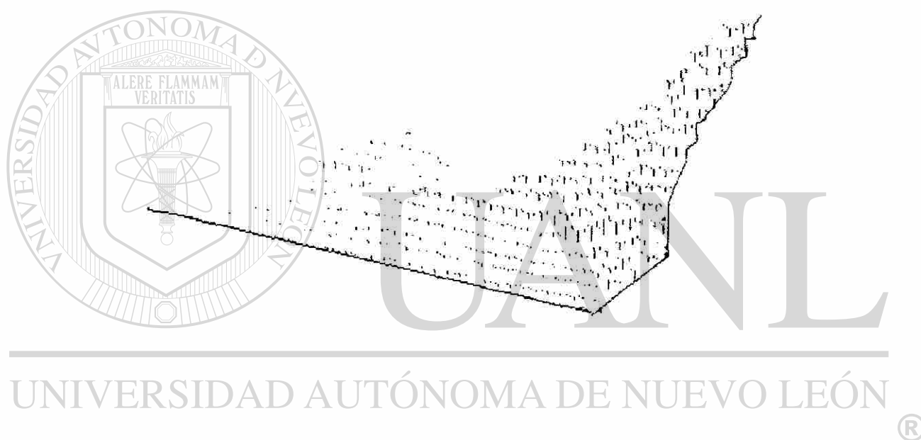
Figura 14. Caracterización de los rasgos topográficos del área de estudio mediante un modelo digital de elevación
