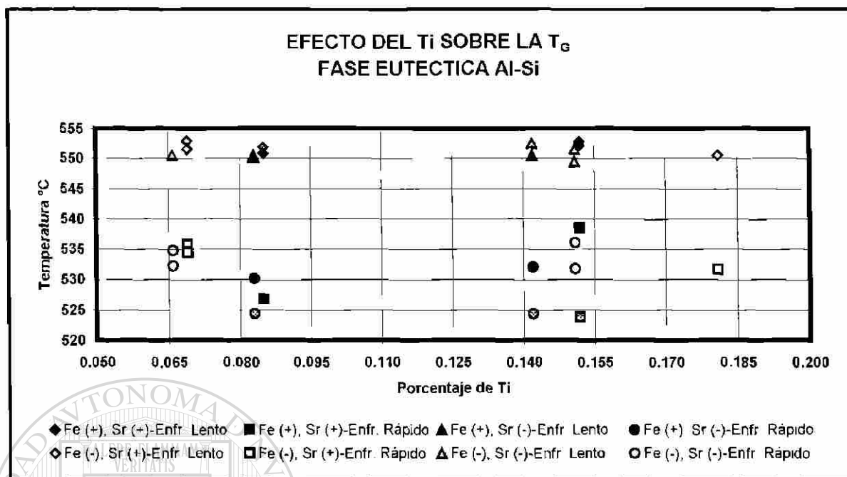
Fig. 5.13g Efecto de la concentración de Ti en la T_G en la solidificación del eutéctico principal Al-Si
