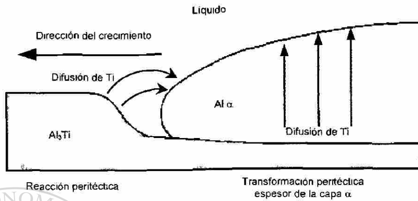
Fig. 2.15 La reacción peritética y su subsecuente transformación [7]
