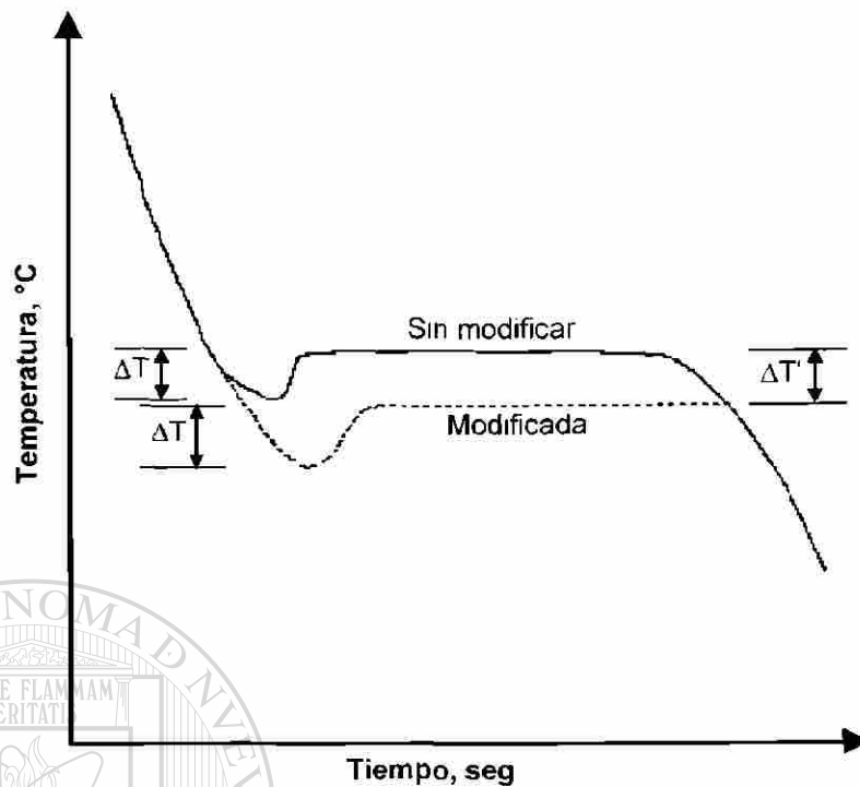
Fig. 3.9 Comparación de dos regiones eutécticas en la curva de enfriamiento entre una aleación modificada y sin modificar [5]
