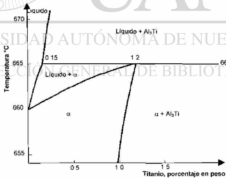
Fig. 2.12 Detalle del diagrama de fase Al-Ti Indicando el punto peritético a 665°C y a 0.15% de titanio [7]
