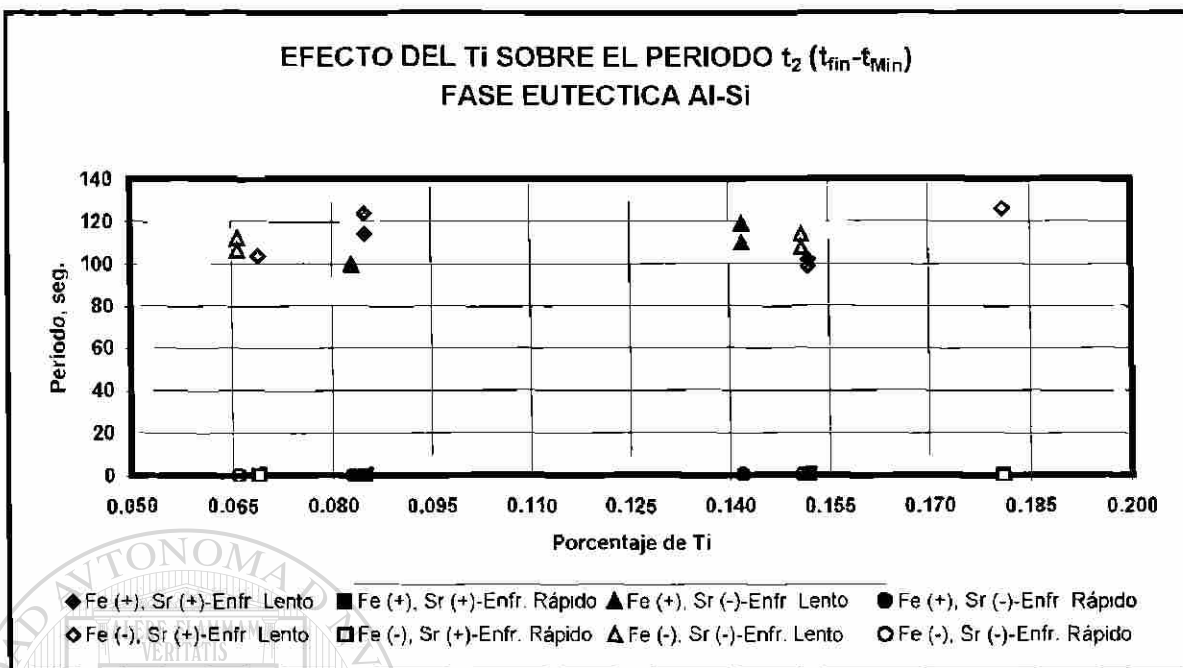
Fig. 5.13c Efecto de la concentración de Ti en el periodo t_2 en la solidificación del eutéctico principal Al-Si
