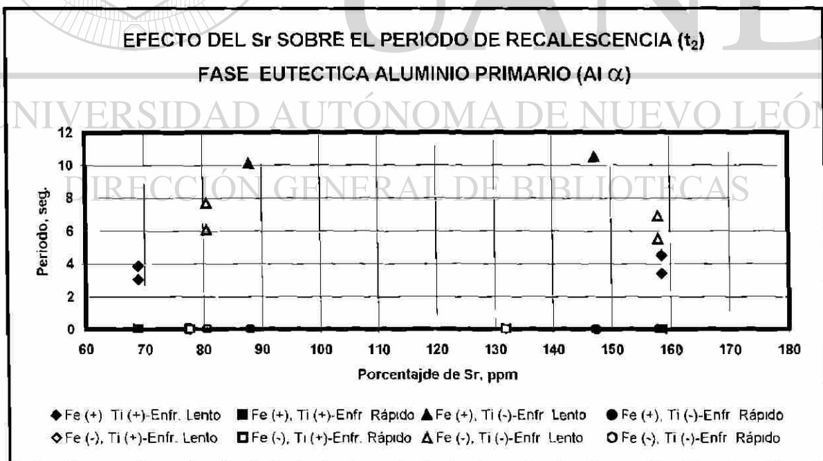
Fig. 5.10c Efecto de la concentración de Sr en el período de recalentamiento en la solidificación de aluminio primario
