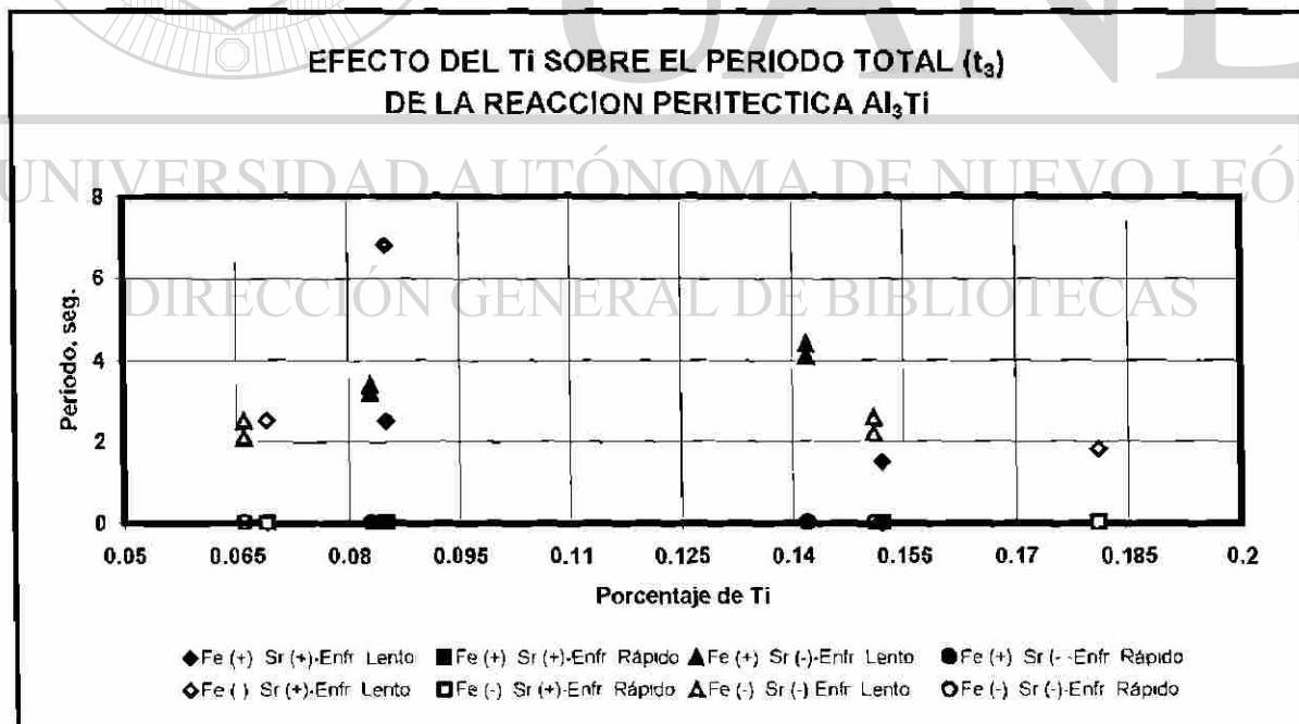
Fig. 5.5b Efecto de la concentración de Ti en el periodo total de la reacción peritética Al_3Ti
