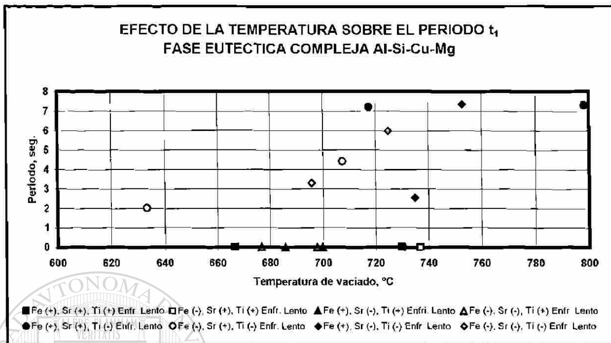
Fig. 5.15a Efecto de la temperatura de vaciado en el período t_1 en la solidificación del eutéctico complejo Al-Si-Cu-Mg
