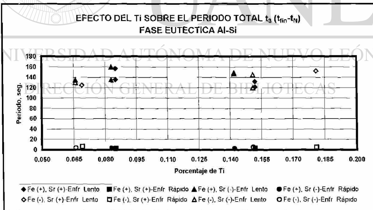
Fig. 5.13d Efecto de la concentración de Ti en el periodo total t_3 en la solidificación del eutéctico principal Al-Si
