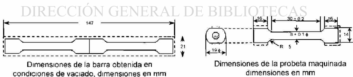
Fig. 4.6 Dimensiones de la barra obtenida y plano de probeta maquinada para la realización de los ensayos mecánicos
