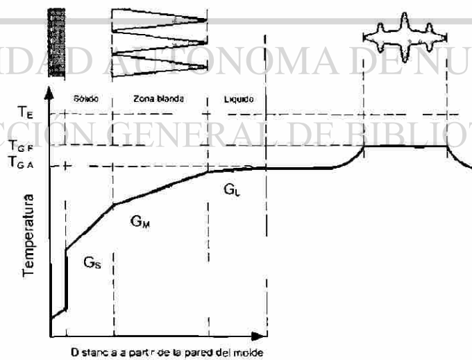
Fig. 2.6 Distribución de temperaturas durante la solidificación de un cristal [7]
