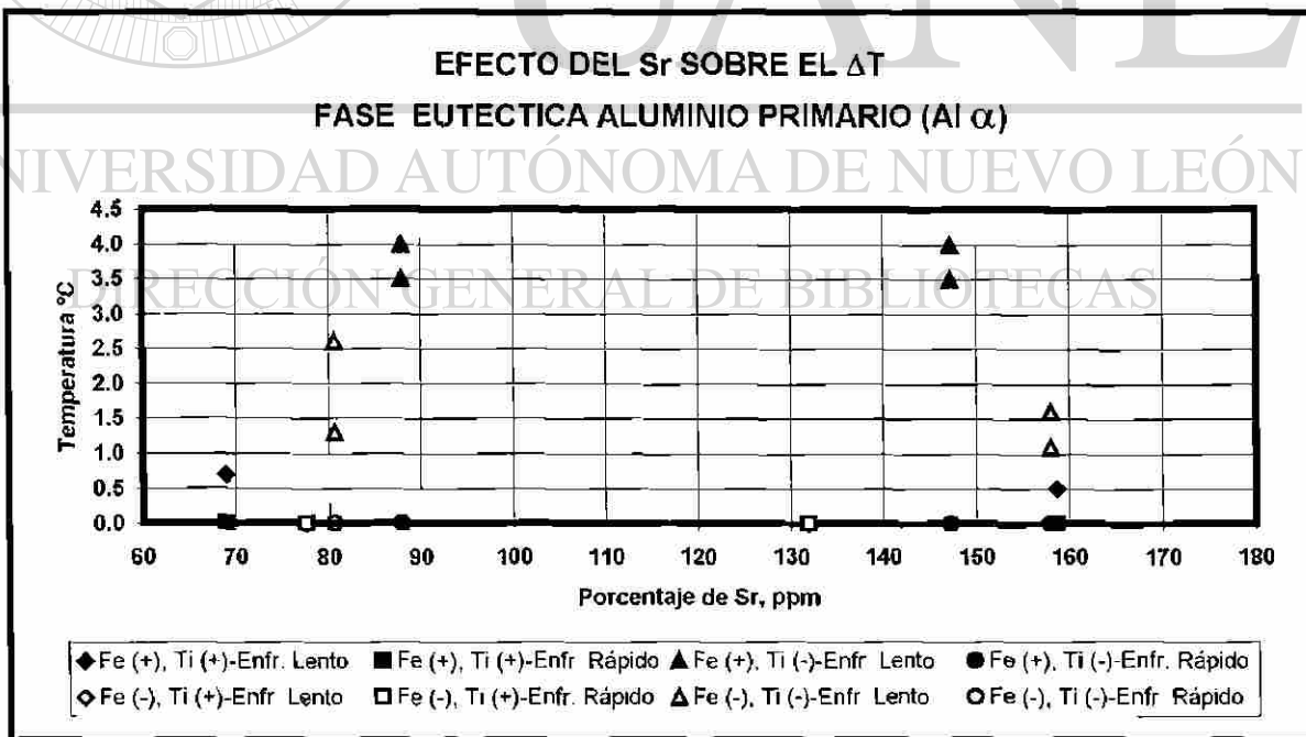
Fig. 5.10a Efecto de la concentración de Sr en el Subenfriamiento ( \Delta T ) en la solidificación de aluminio primario
