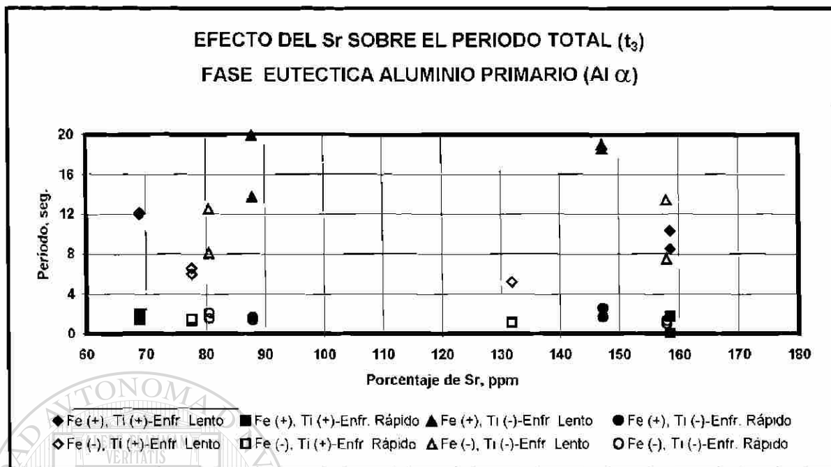
Fig. 5.10d Efecto de la concentración de Sr en el período total en la solidificación de aluminio primario
