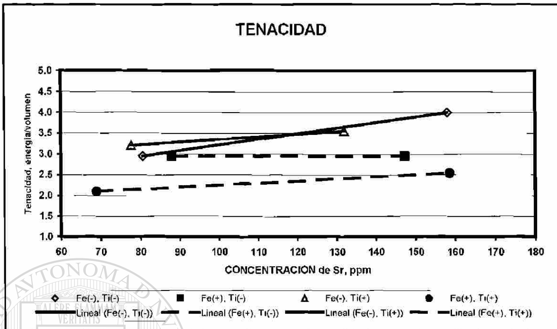
Fig. 5.22e Efecto de la concentración de Sr en la tenacidad para las diferentes aleaciones
