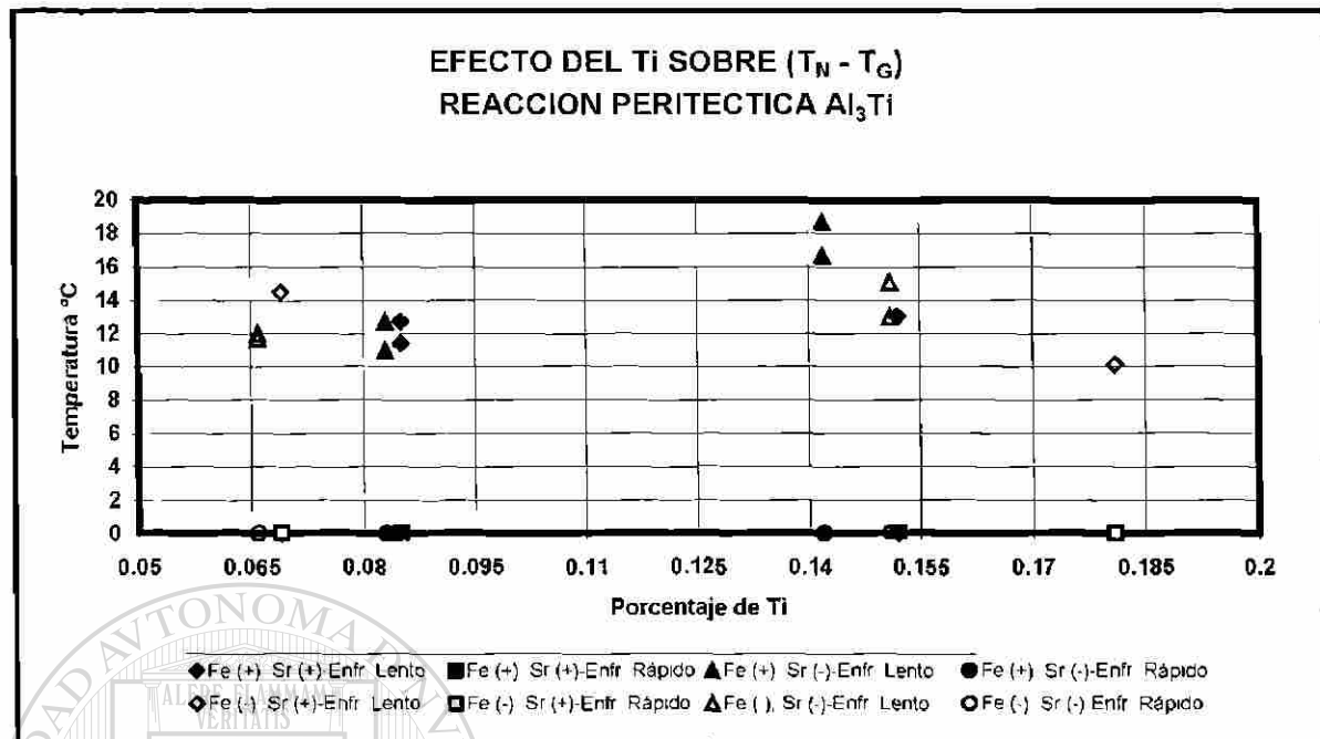
Fig. 5.5a Efecto de la concentración de Ti en T_N - T_G de la reacción peritética Al_3Ti
