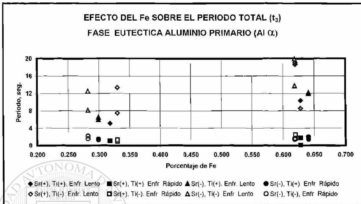
Fig. 5.8d Efecto de la concentración de Fe en el período total en la solidificación de aluminio primario
