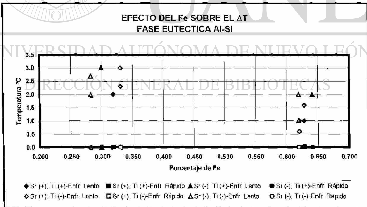
Fig. 5.12a Efecto de la concentración de Fe en el subenfriamiento ( \Delta T ) en la solidificación del eutéctico principal Al-Si
