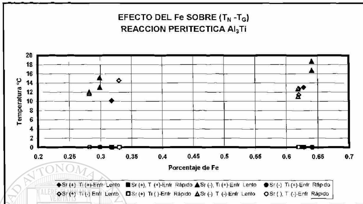
Fig. 5.4a Efecto de la concentración de Fe en la diferencia (T_N - T_G) de la reacción peritética Al_3Ti
