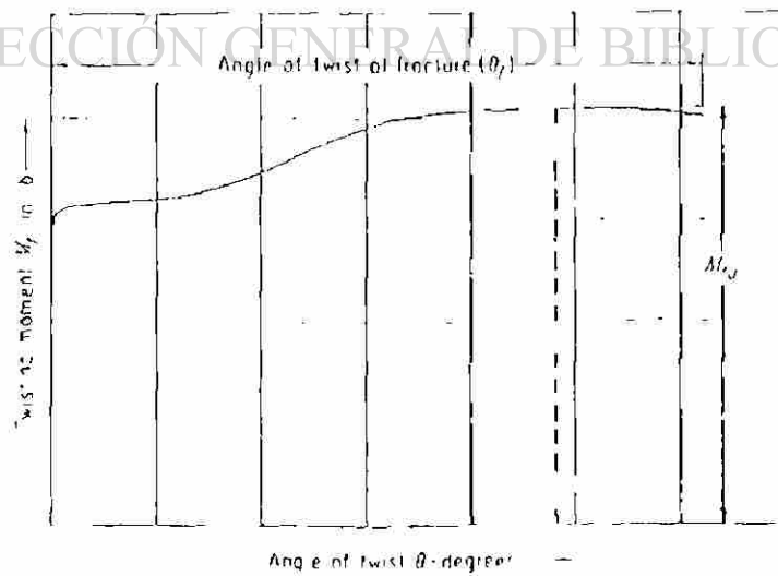
Fig 4.3 Obtención de la tenacidad
